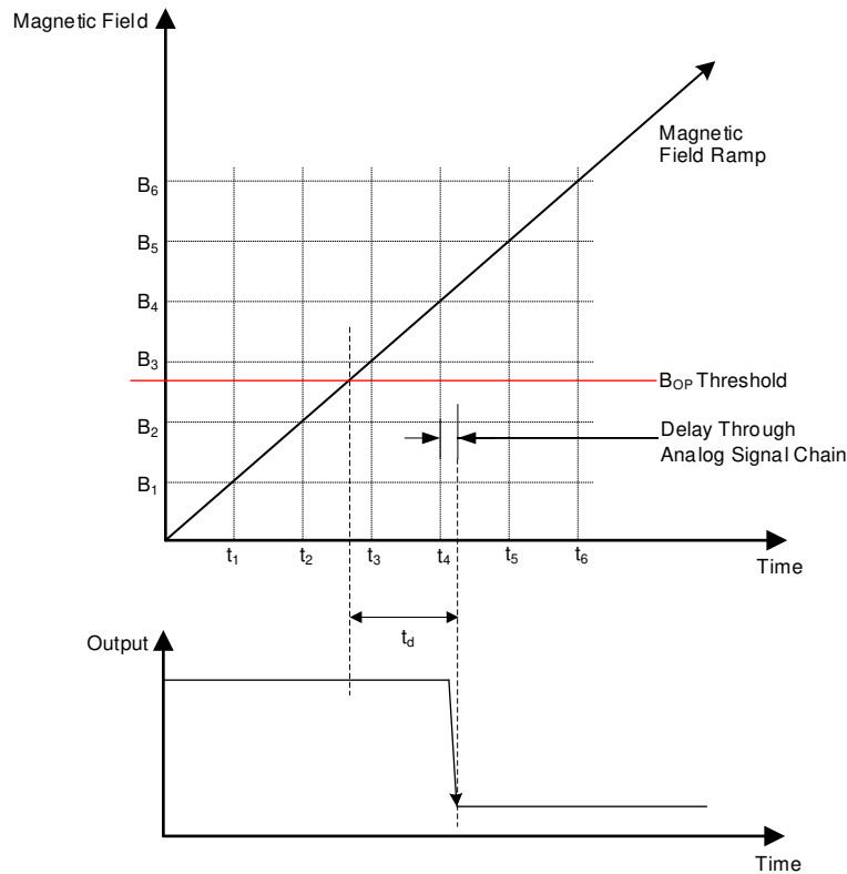
图 18. Propagation Delay
