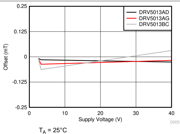
图 6-9. 偏移与 V_{CC} 之间的关系
