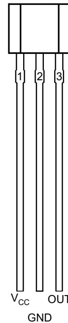
图 5-2. LPG 封装 3 引脚 TO-92 顶视图
