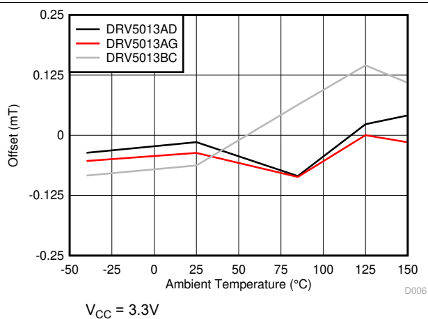
图 6-10. 偏移与温度之间的关系
