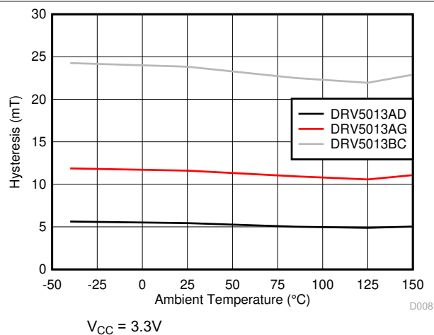
图 6-8. 迟滞与温度之间的关系
