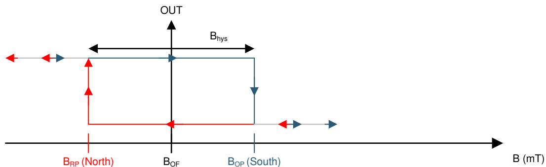
图 7-2. DRV5013-Q1 - B_{OP} > 0
