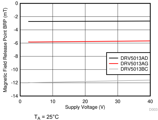
图 6-5. B_{RP} 与 V_{CC} 之间的关系
