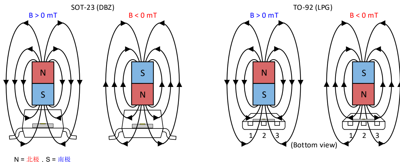
图 7-1. 场方向定义
