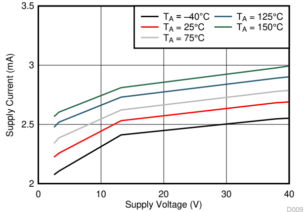
图 6-1. I_{CC} 与 V_{CC} 之间的关系
