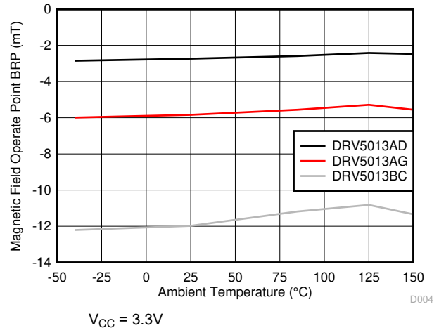
图 6-6. B_{RP} 与温度之间的关系
