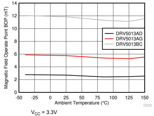
图 6-4. B_{OP} 与温度之间的关系
