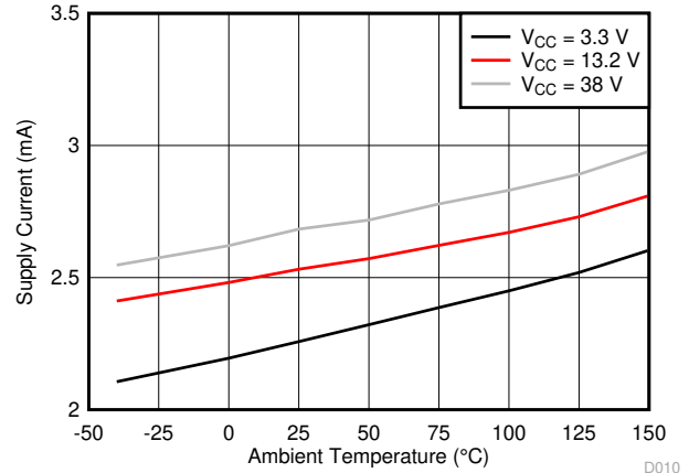
图 6-2. I_{CC} 与温度之间的关系
