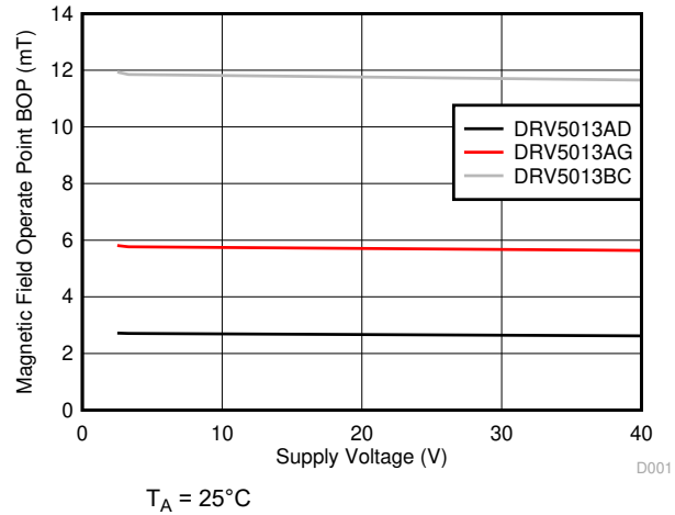
图 6-3. B_{OP} 与 V_{CC} 之间的关系
