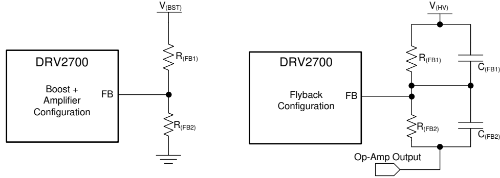
图 8-3. External Network
