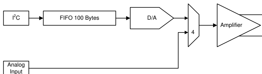
图 7-1. Front-End Interface
