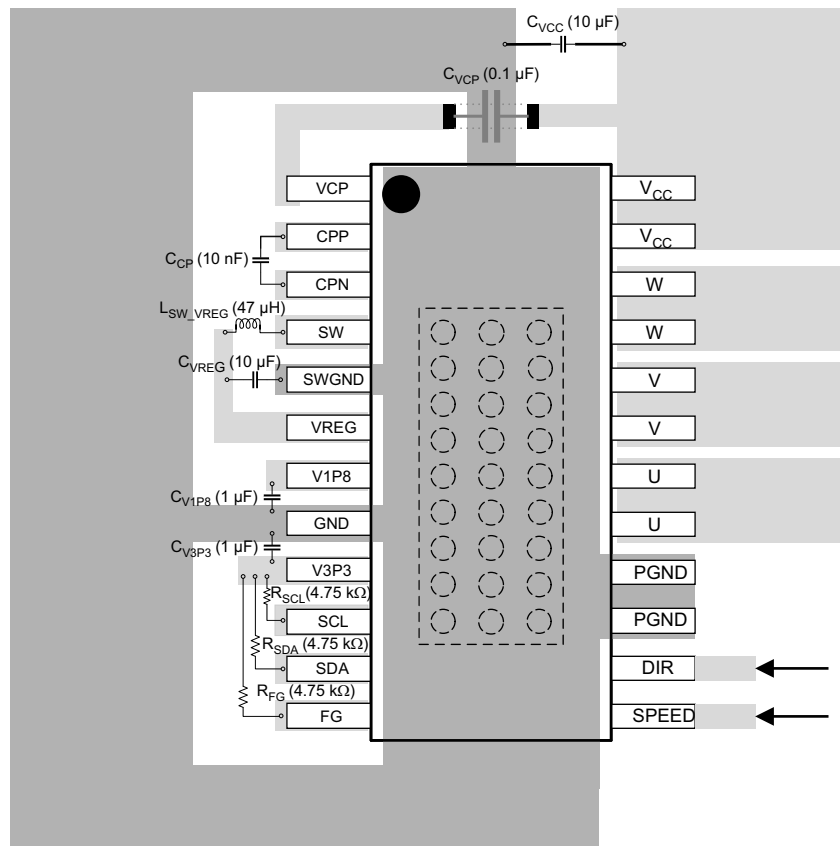
图 11-1. Layout Diagram
