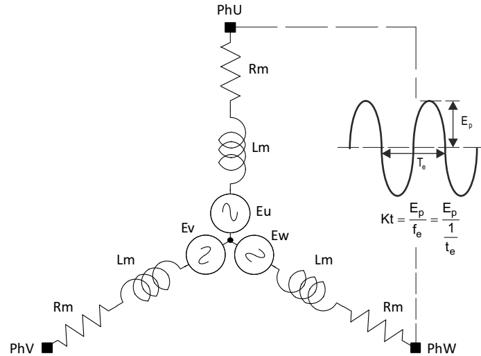
图 8-9. K_{tPH} Definition
