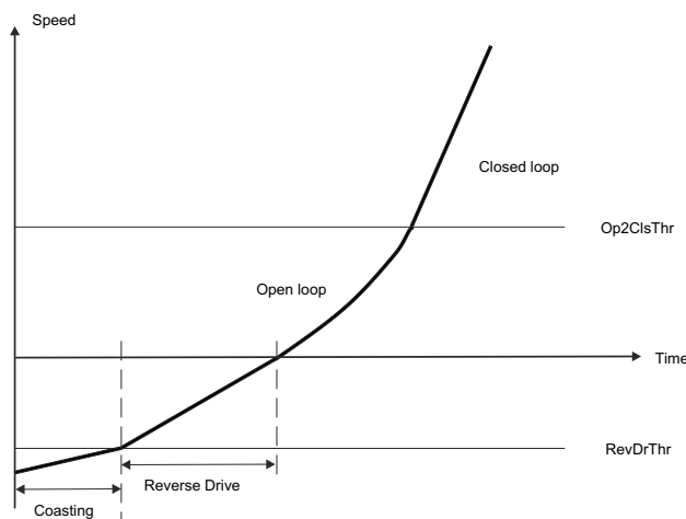
图 8-13. Reverse Drive Function
