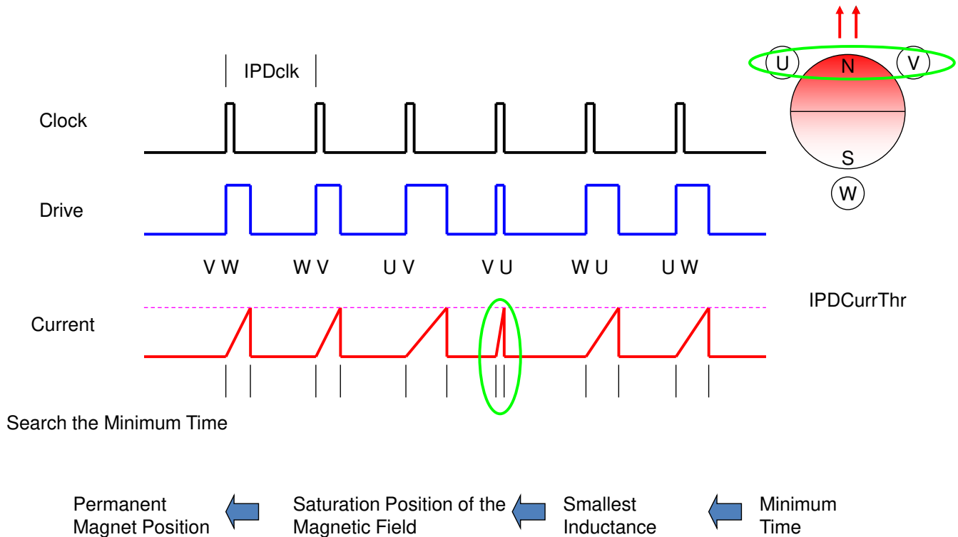
图 8-14. IPD Function
