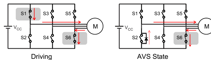
图 8-35. Inductive AVS
