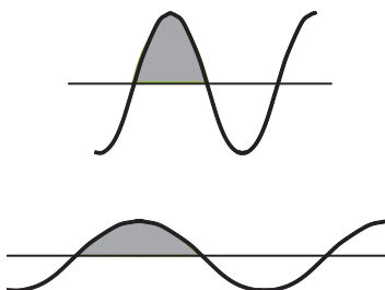
图 31. BEMF Integration
