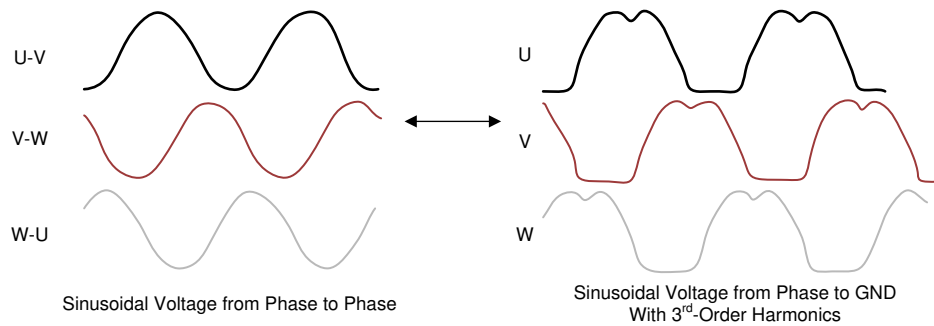
图 7-2. Sinusoidal Voltage
