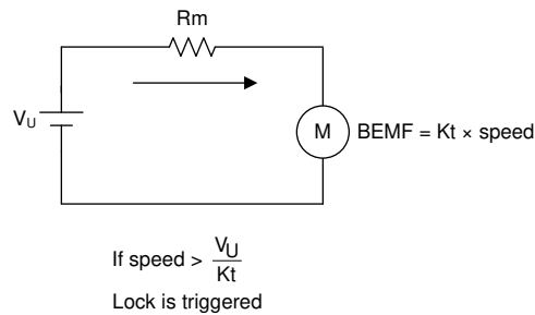
图 7-11. BEMF Monitoring
