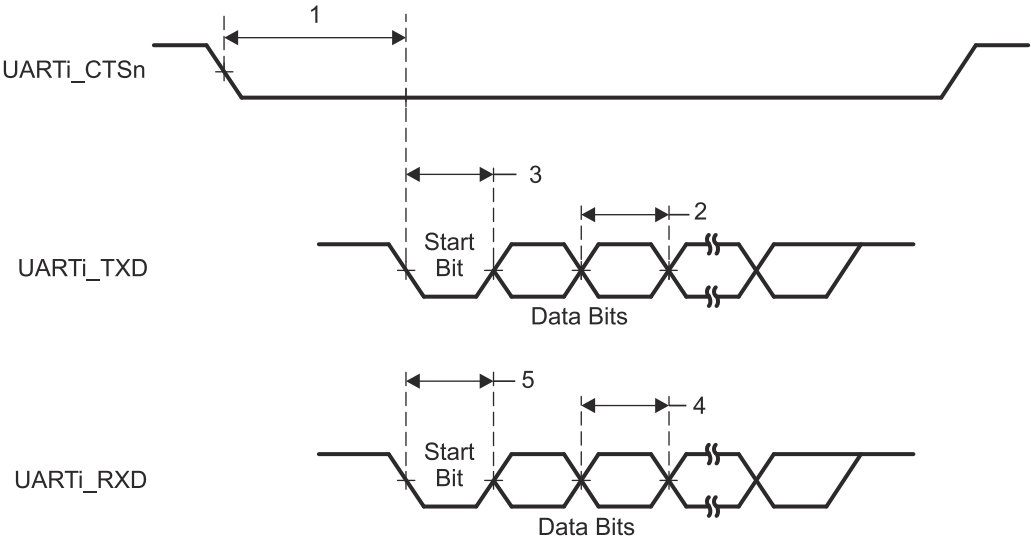
图 6-120. UART Timing
