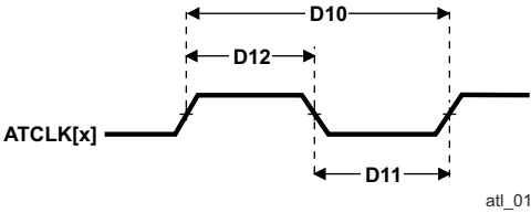
图 6-38. ATCLK[x] Timing
