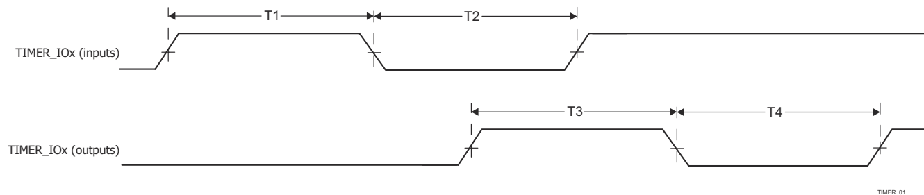
图 6-119. Timer Timing
