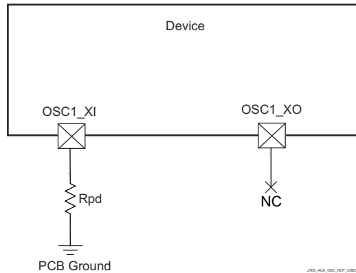
图 6-33. OSC1 Not Used
