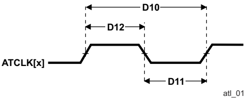
图 6-38. ATCLK[x] Timing
