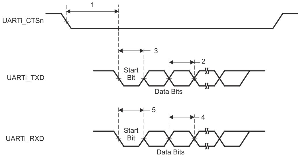
图 6-120. UART Timing
