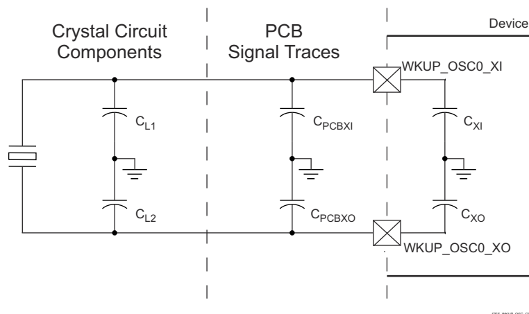
图 7-26. Load Capacitance
