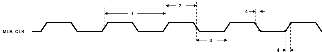
图 5-77. MLB_CLK Timing
