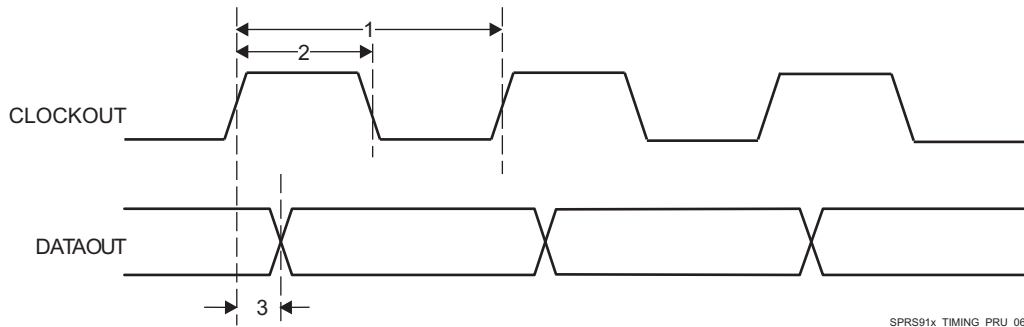
图 5-114. PRU-ICSS PRU Shift Out Timing
