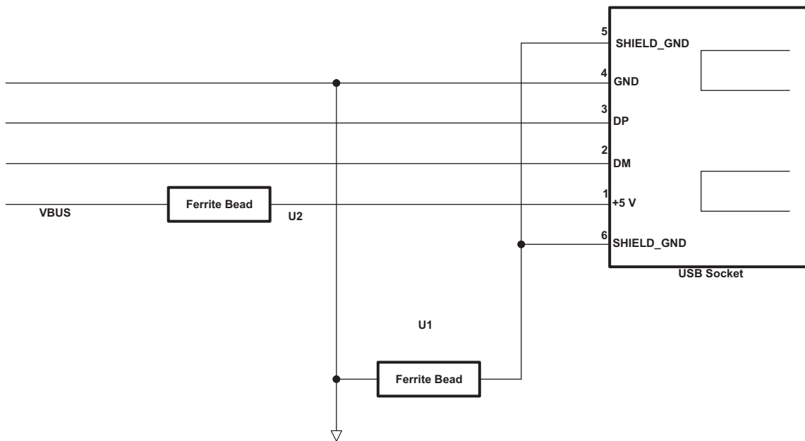
图 7-23. USB Connector
