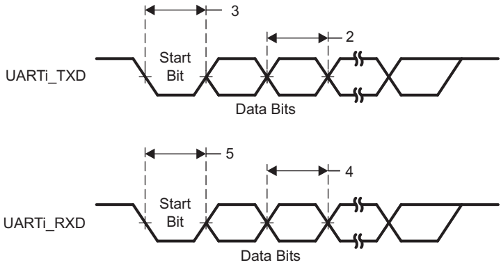
图 5-48. UART Timing
