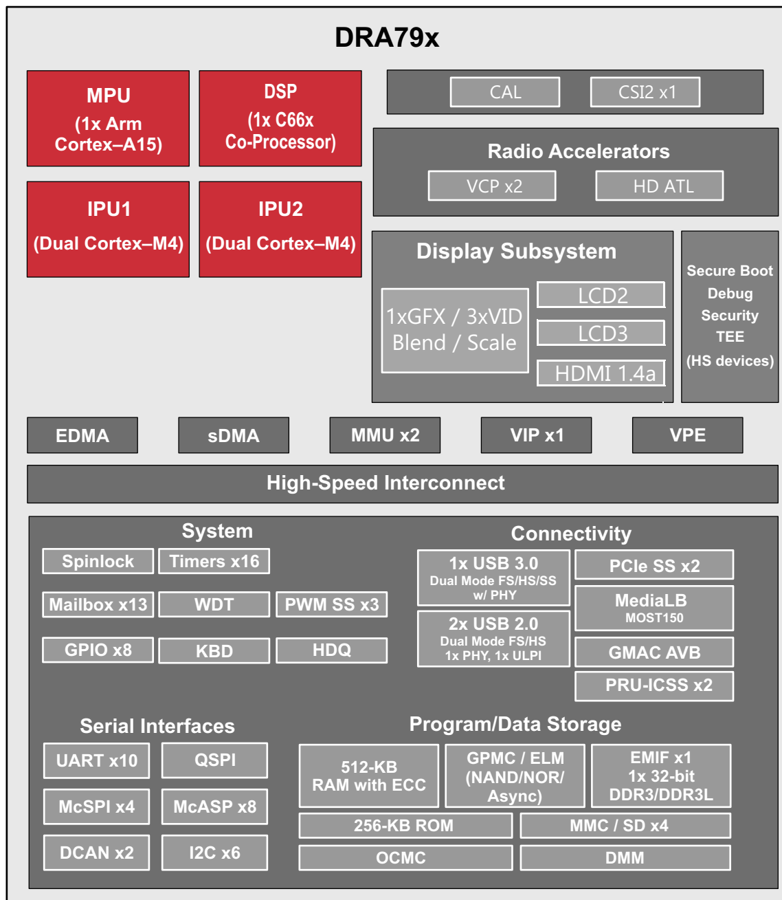
图 1-1. DRA79x 方框图
