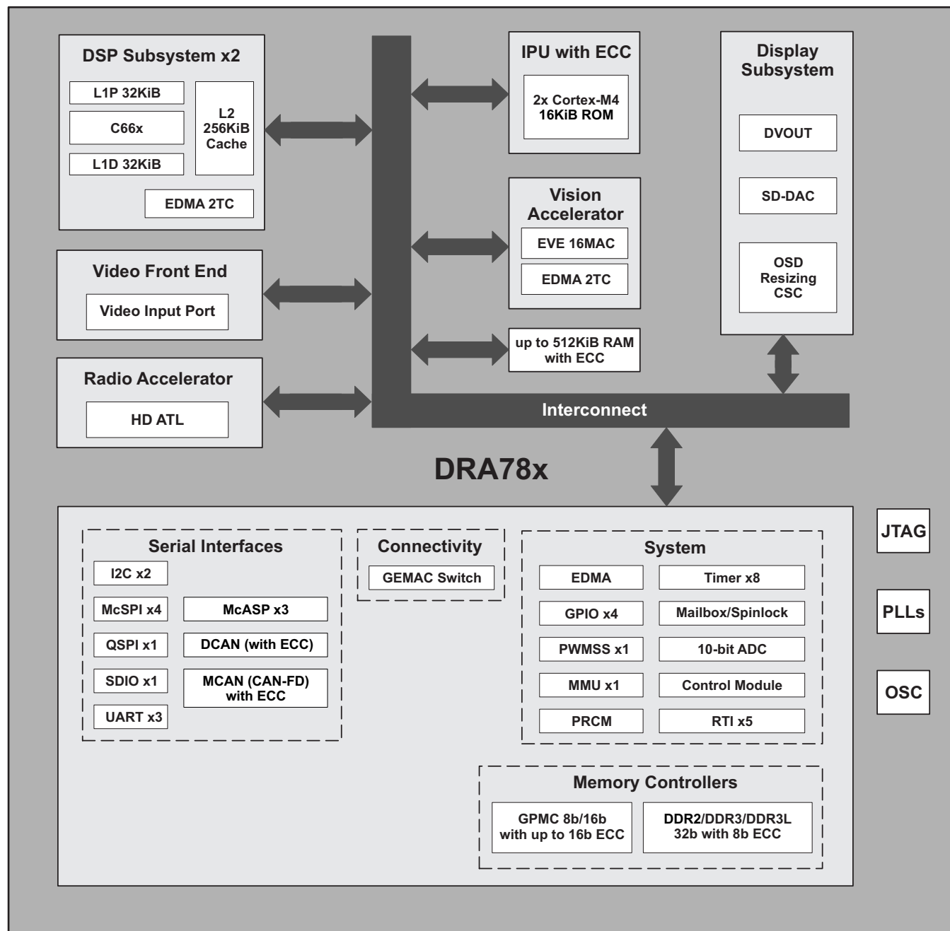
图 1-1. DRA78x 框图
