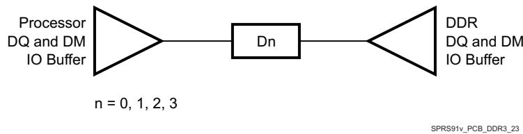
图 7-52. DQ/DM Topology
