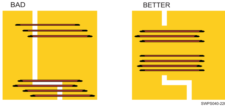
图 7-17. Trace Examples
