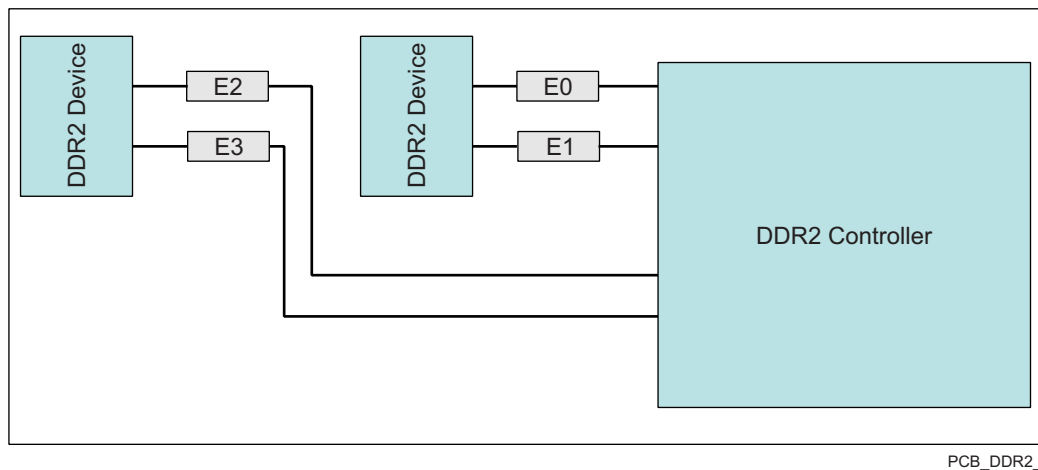
图 7-53. DQS and DQ Routing and Topology
