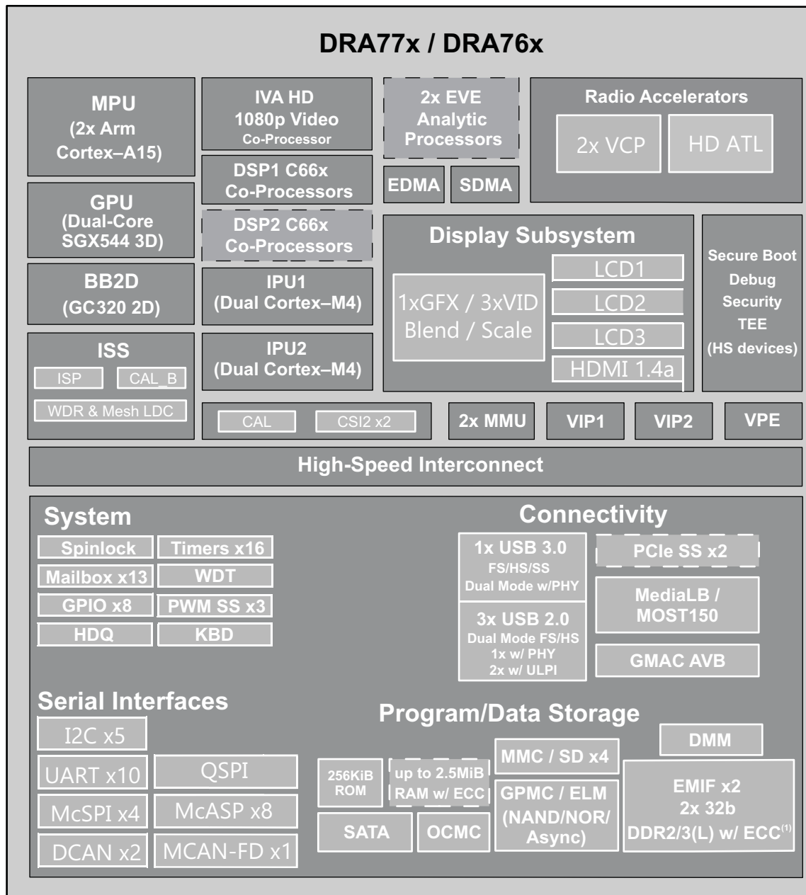
图 1-1. DRA77xP、DRA76xP 方框图
