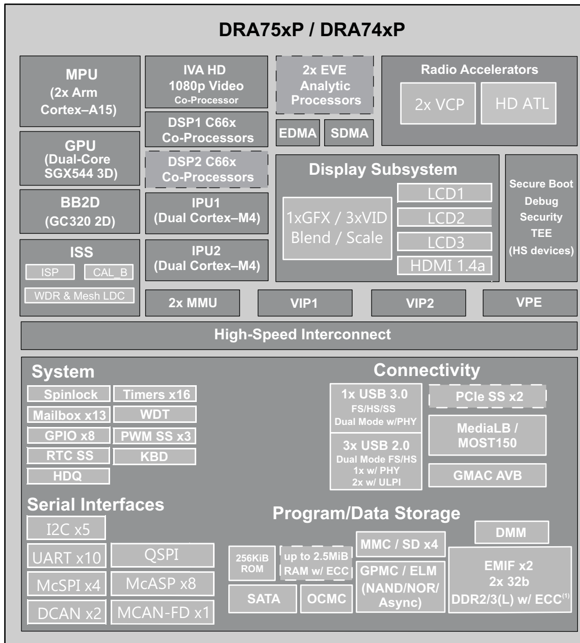
图 1-1. DRA75xP、DRA74xP 方框图
