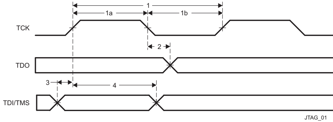
图 5-115. JTAG Timing
