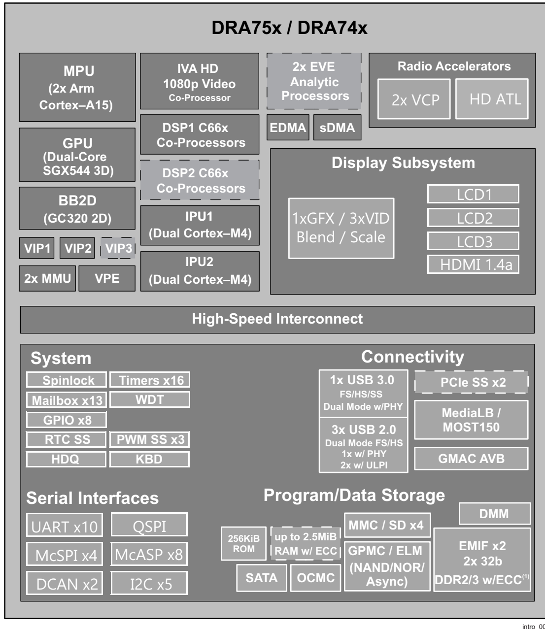
图 1-1. DRA75x、DRA74x 方框图
