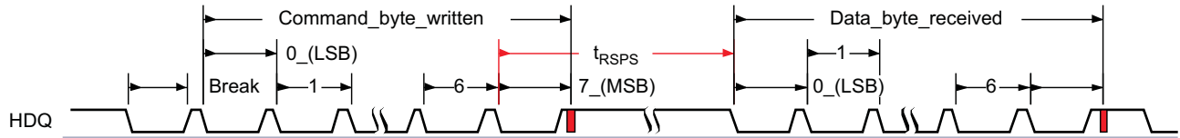
图 7-28. HDQ Communication Timing
