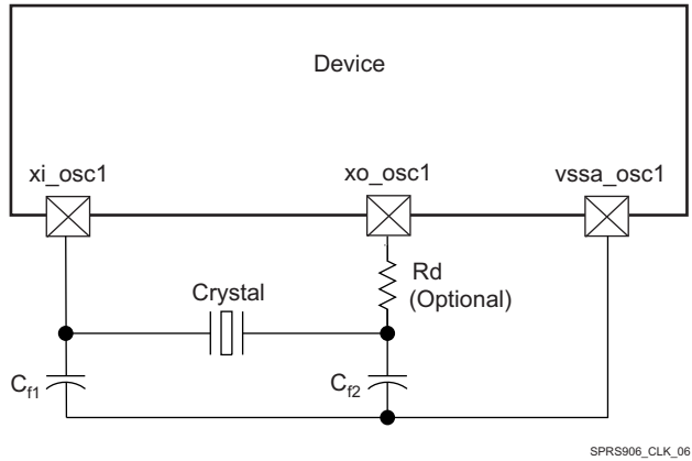
图 6-6. Crystal Implementation
