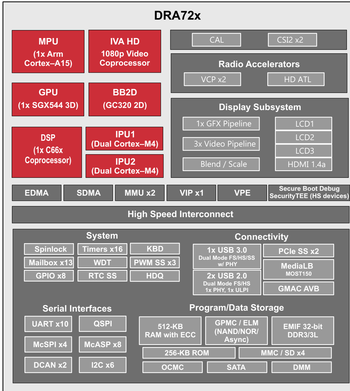
图 1-1. DRA72x 方框图
