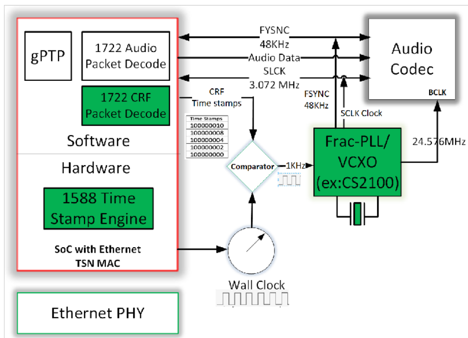
图 5-2. 典型的以太网音频架构
