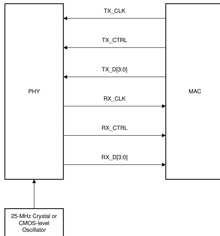
图 7-13. RGMII 连接
