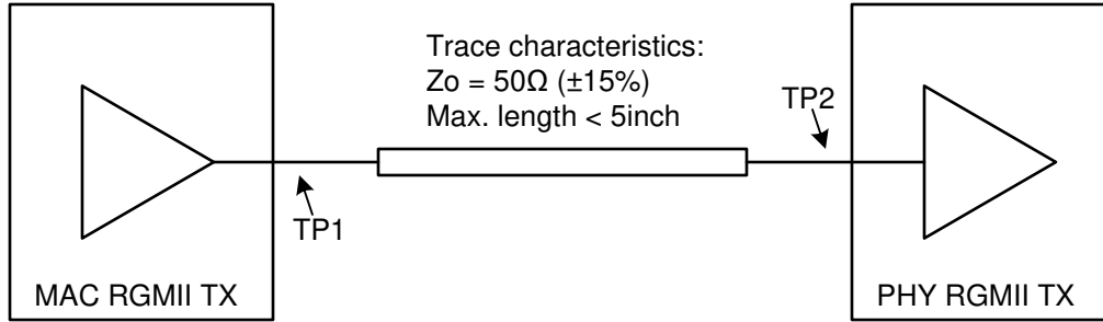
图 7-14. RGMII TX 要求
