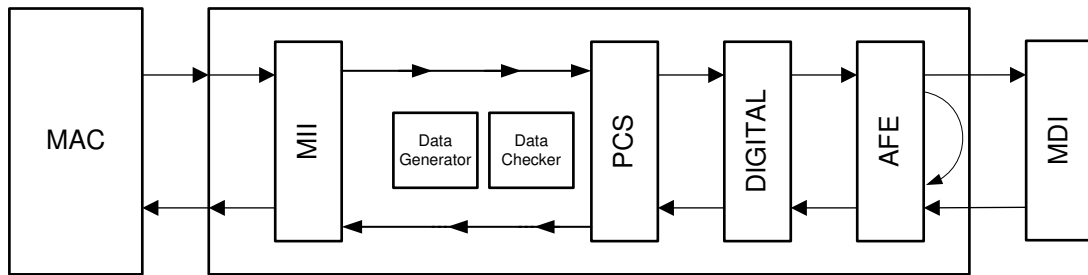
图 7-2. 所有环回
