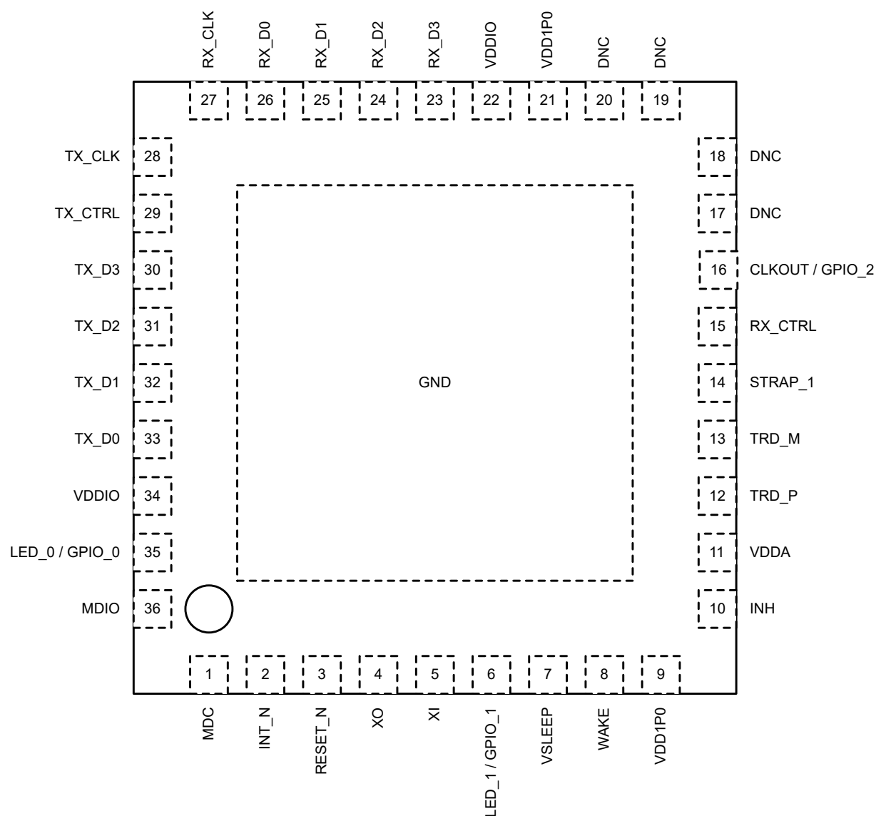
图 5-1. RHA 封装 36 引脚 VQFN 俯视图
