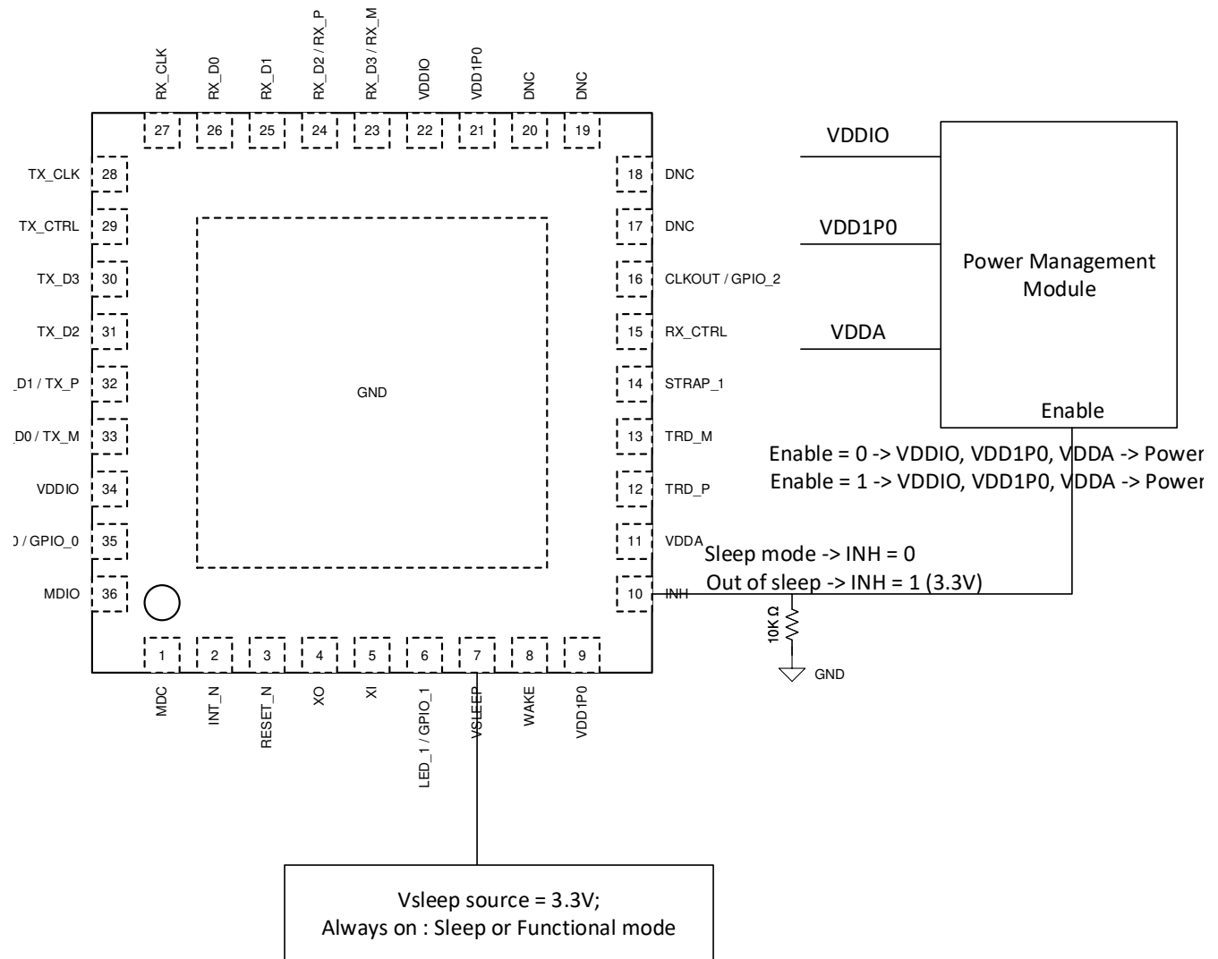
图 7-12. 睡眠模式所需实现
