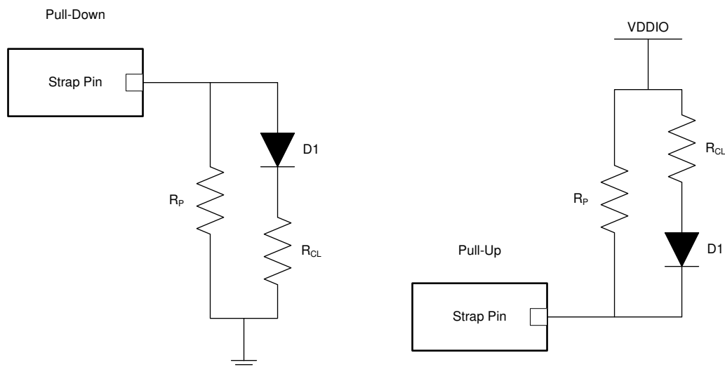
图 7-17. Strap 配置连接示例
