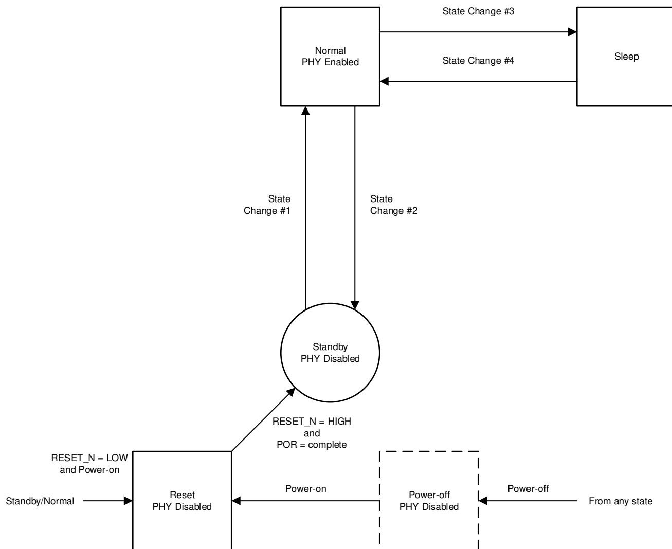
图 7-11. PHY 运行状态图
