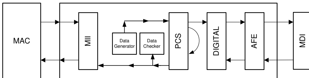
图 7-7. 具有内置数据生成器的 PCS 环回
