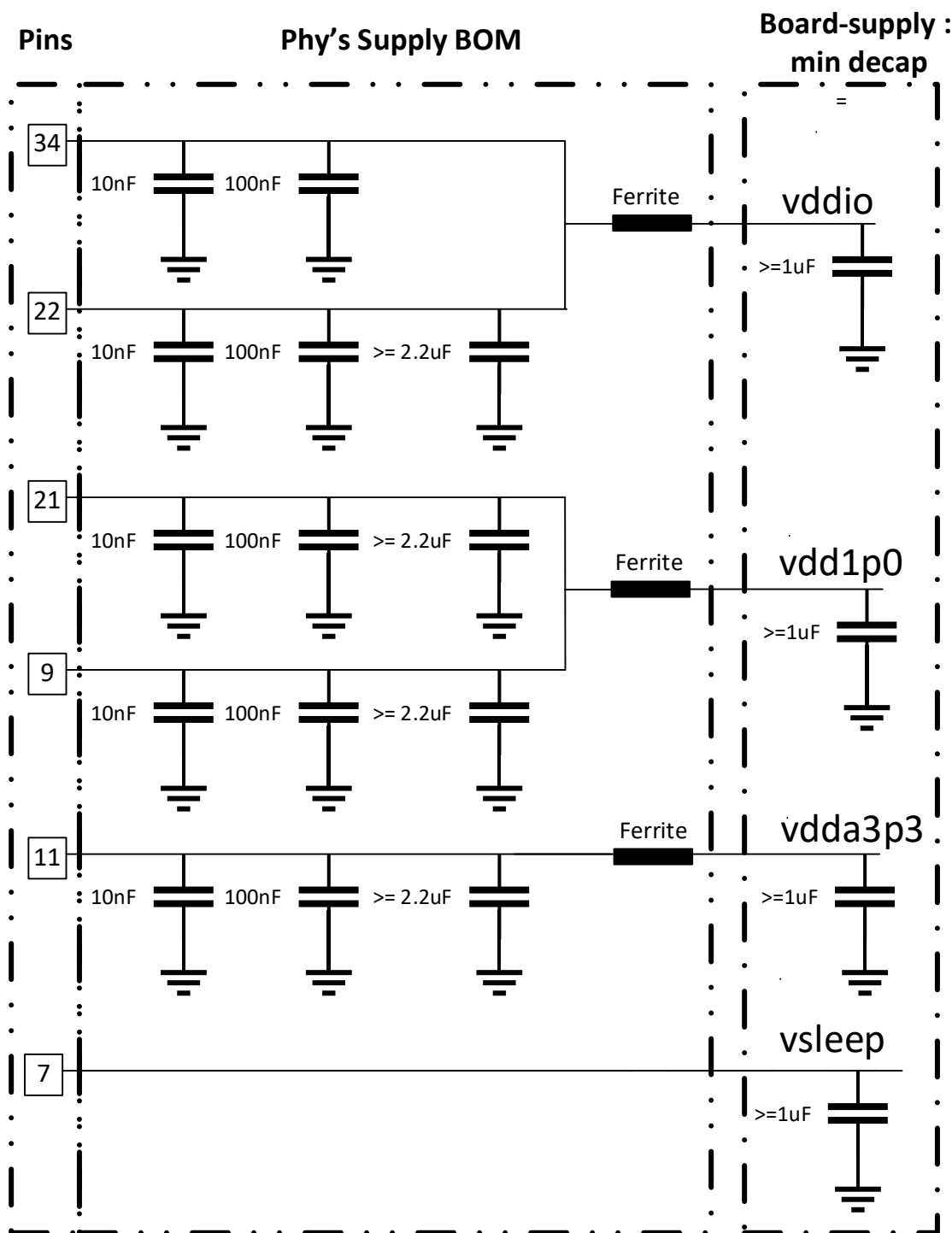
图 8-2. 建议电源去耦网络 (如果应用采用睡眠模式)
