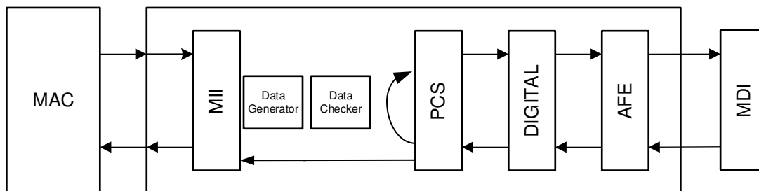
图 7-10. 具有外部数据生成器的 xMII 反向环回
