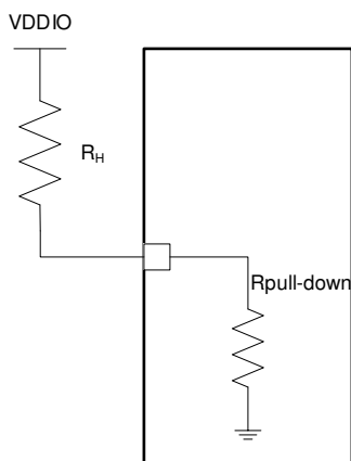
图 7-16. 配置 (Strap) 电路
