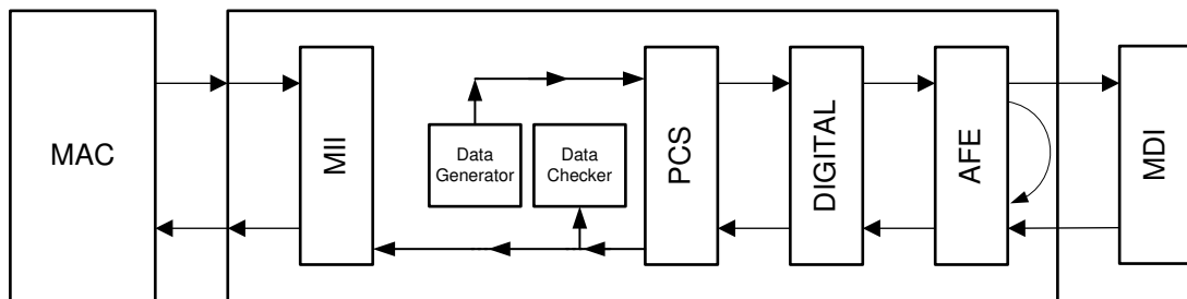
图 7-3. 具有内置数据生成器的模拟环回
