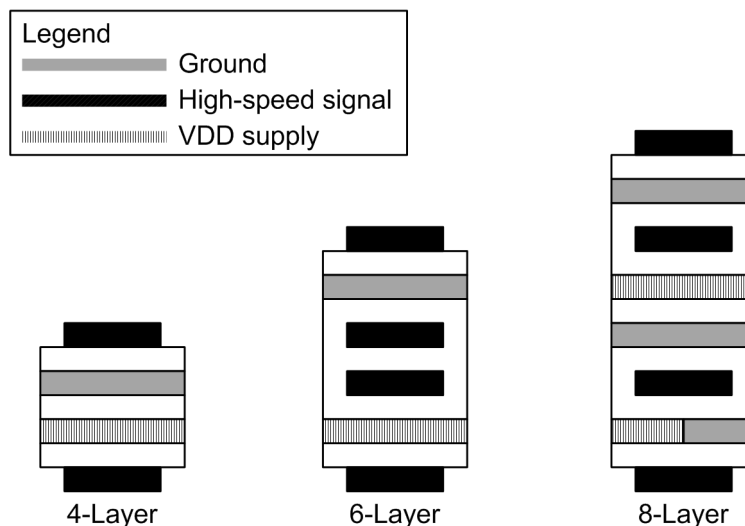
图 8-6. 建议 PCB 层堆叠
