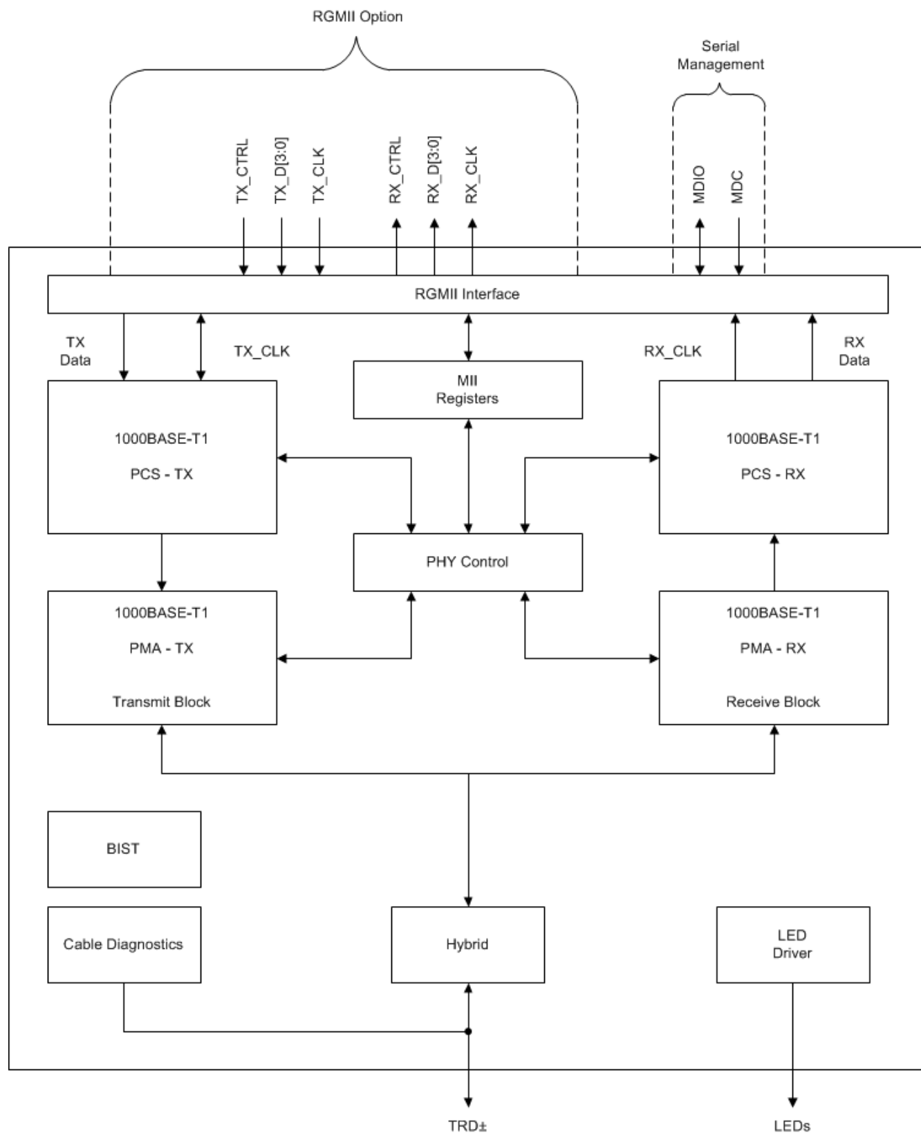
图 7-1. DP83TG720R-Q1 功能方框图
