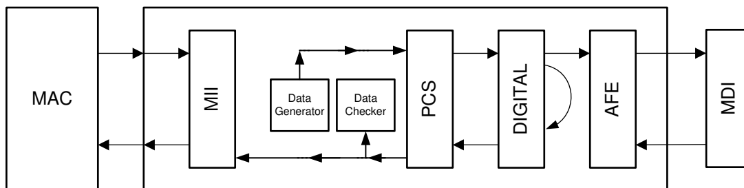
图 7-5. 具有内置数据生成器的数字环回
