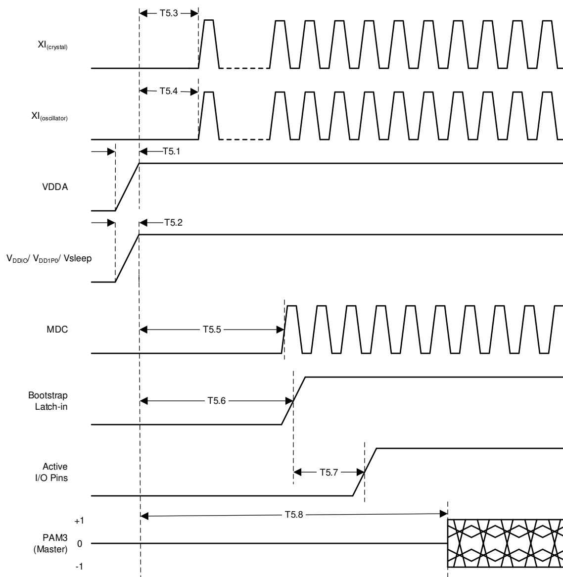
图 6-1. 上电时序
