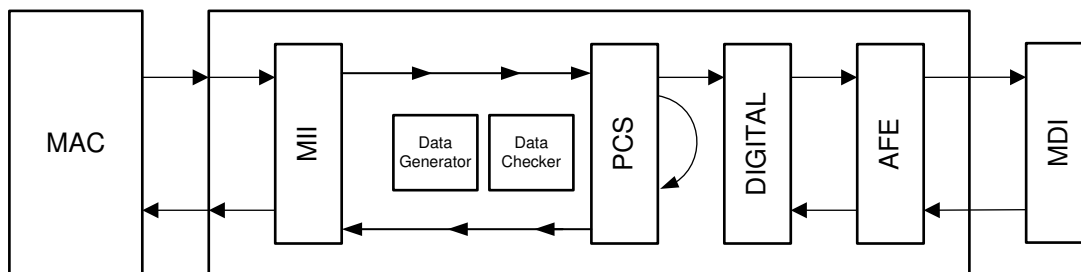
图 7-8. 具有外部数据生成器的 PCS 环回
