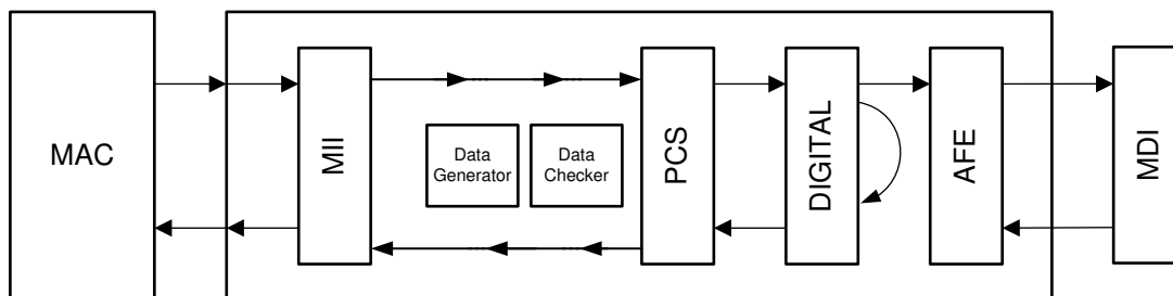
图 7-6. 具有外部数据生成器的数字环回
