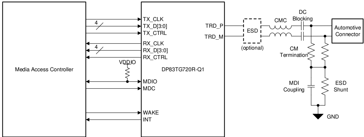
图 8-1. 典型应用 (RGMII)
