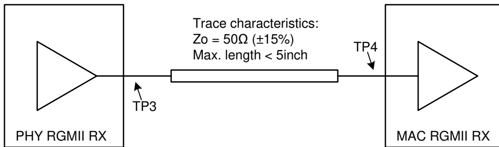
图 7-15. RGMII RX 要求
