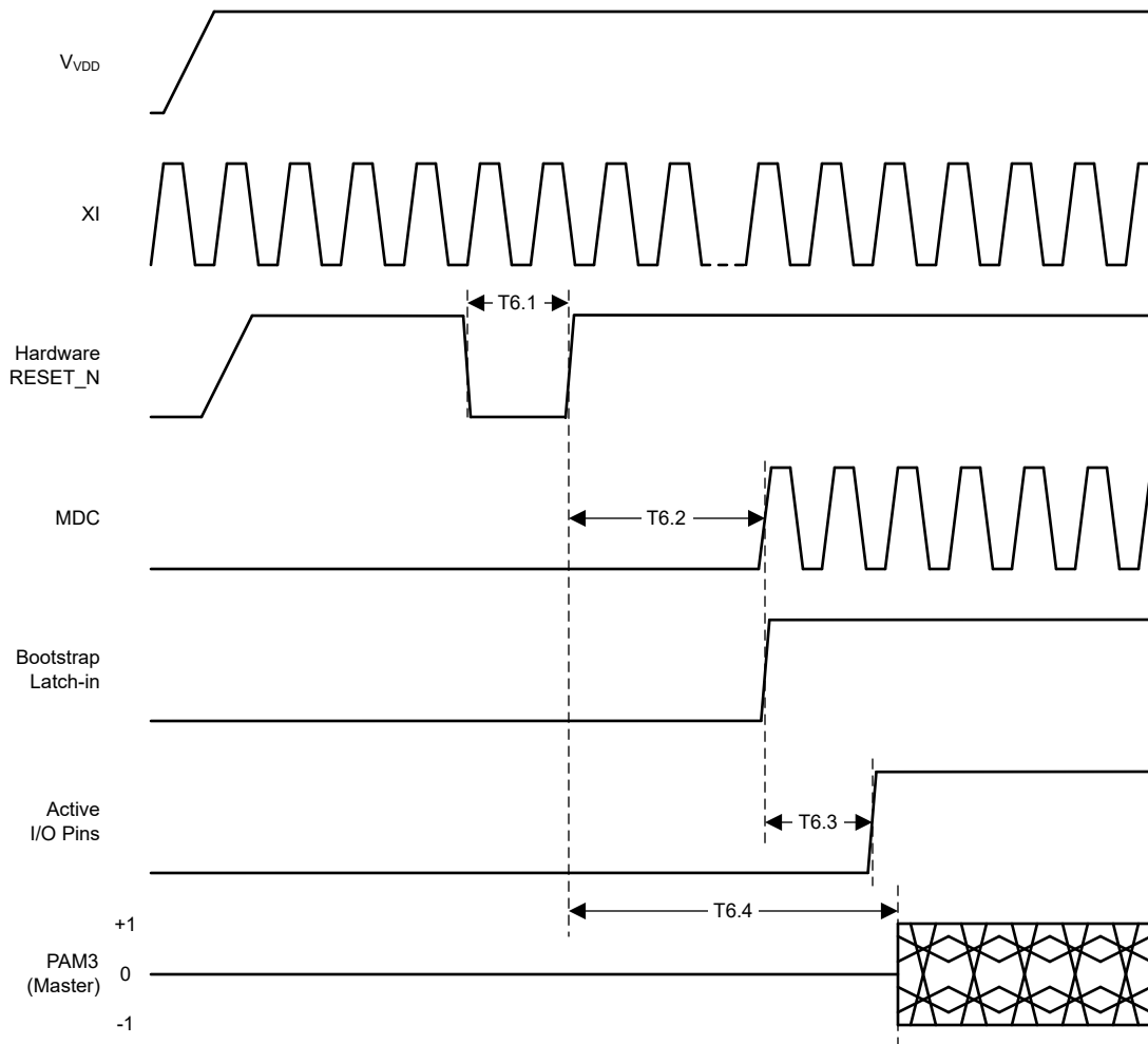
图 7-9. Reset Timing
