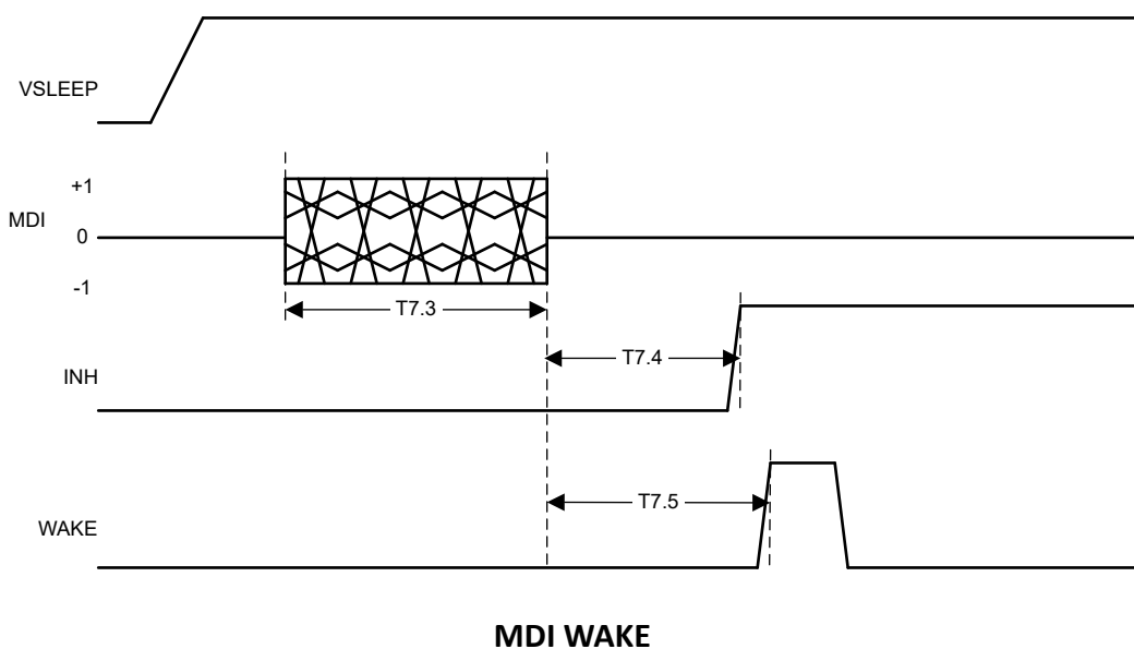
图 6-9. WAKE Timing
