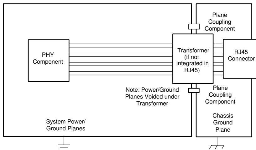
图 8-16. Copper Ethernet Layout Example
