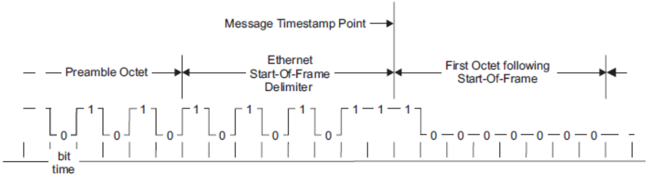
图 7-2. IEEE 1588 Message Timestamp Point
