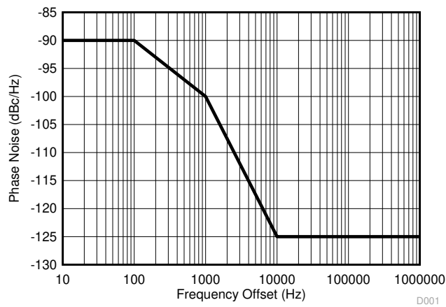
图 8-3. 25MHz Oscillator Phase Noise
