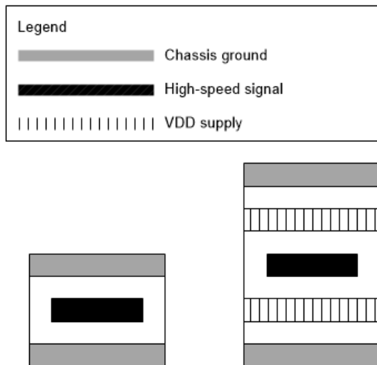
图 8-15. Alternative Layer Stack-Up
