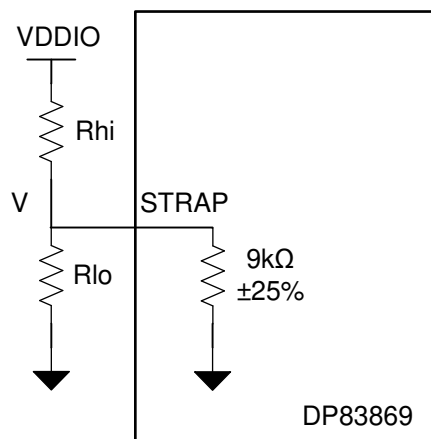
图 7-15. Strap Circuit
