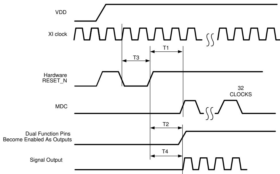
图 6-2. Reset Timing
