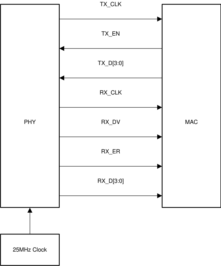
图 7-8. MII Signaling
