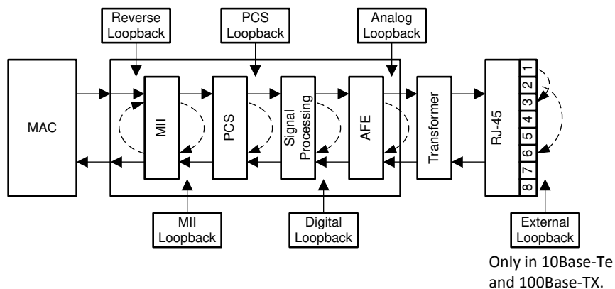
图 7-4. Loopbacks
