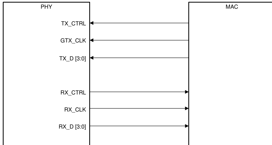
图 7-7. RGMII Connections
