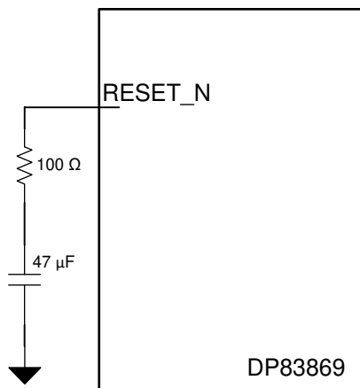
图 7-17. RESET_N Circuit
