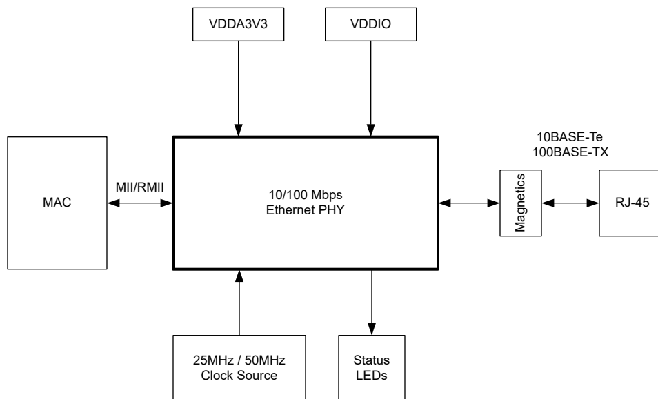
图 9-1. DP83826 典型应用
