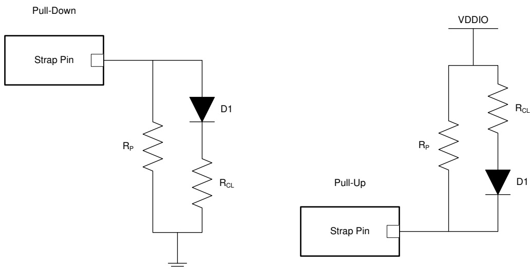
图 8-10. LED 配置 (Strap) 连接示例
