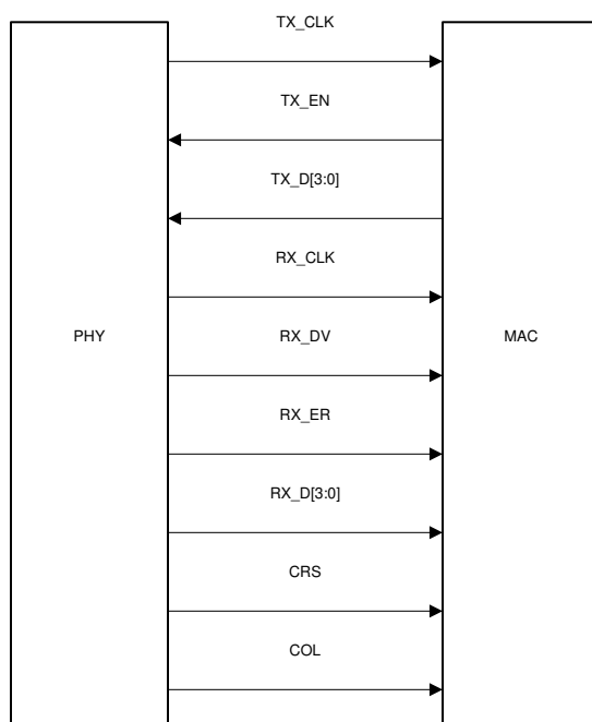
图 8-4. MII 信号
