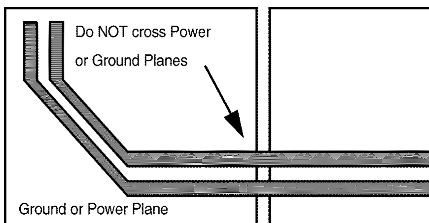
图 9-8. 差分信号对和平面交叉
