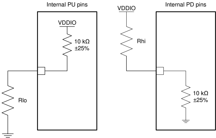
图 8-11. 配置 (Strap) 电路
