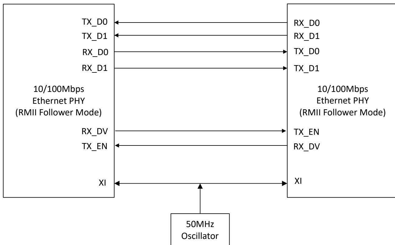
图 8-3. RMII 中继器模式：从-从
