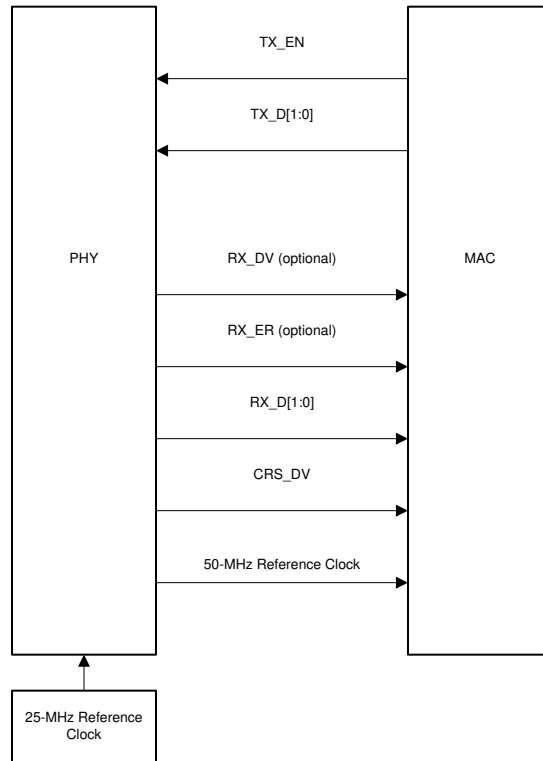
图 8-6. RMII 主信号
