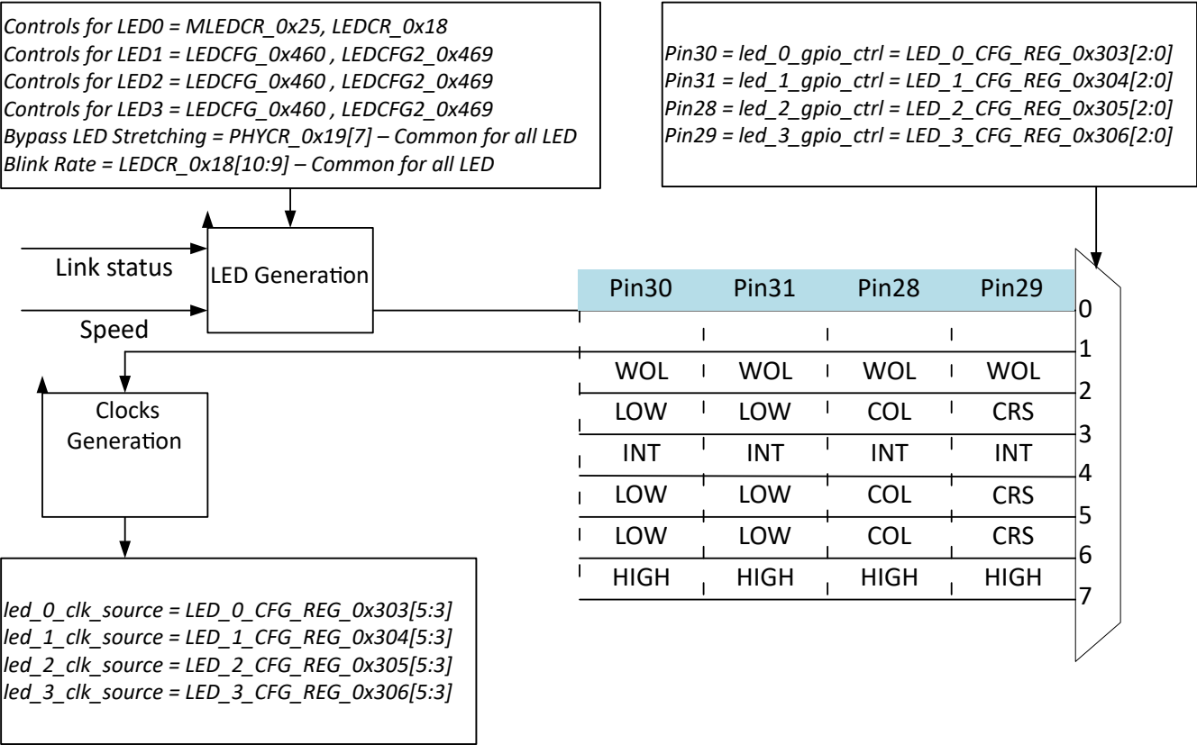
图 8-9. LED 和 GPIO 配置
