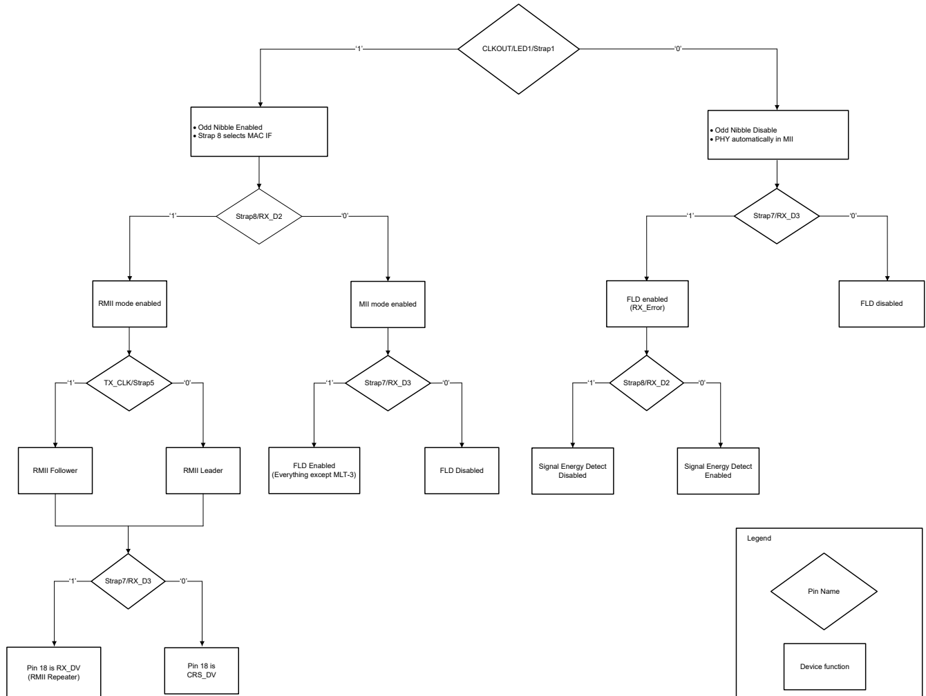
图 8-12. 增强型自动加载流程图
