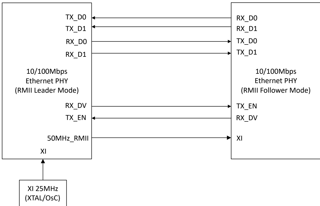
图 8-2. RMII 中继器模式：主-从
