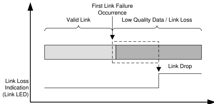
图 8-8. 快速链路丢失
