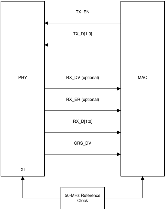
图 8-3. 使用外部 50MHz CMOS 电平振荡器的 RMII 从模式信令
