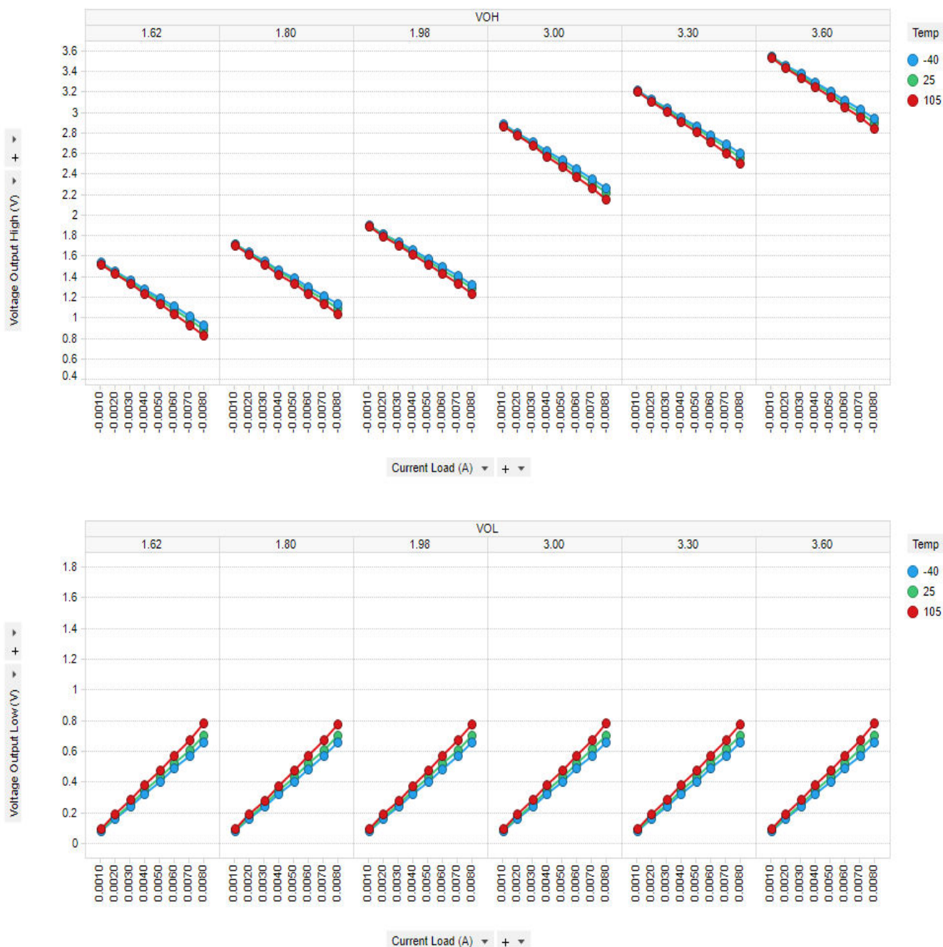
图 9-5. DP83826Ax 输出引脚驱动特性
