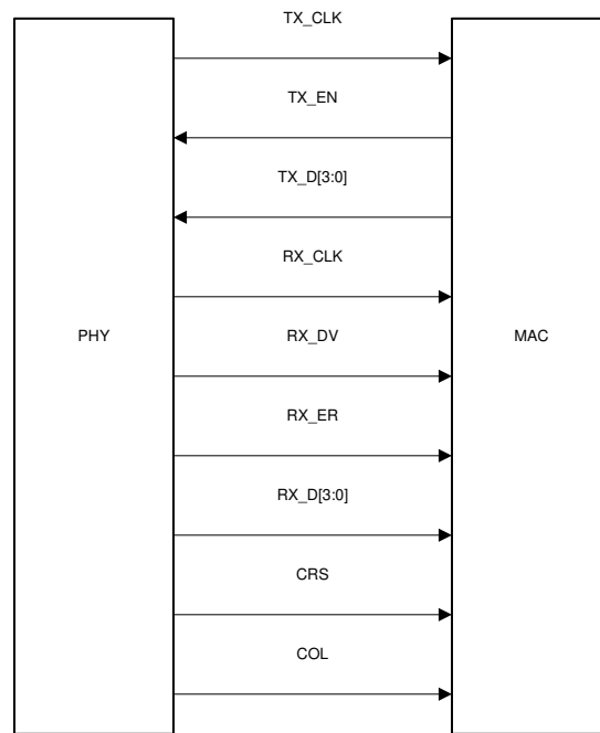
图 8-2. MII 信号
