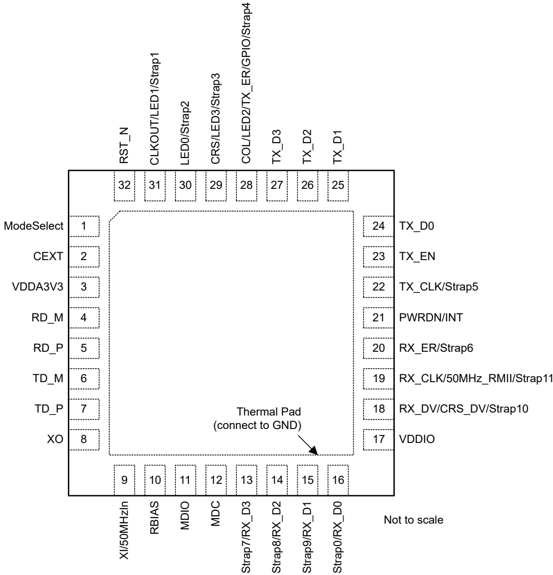
图 5-1. RHB 封装 32 引脚 QFN ( 顶视图 )
