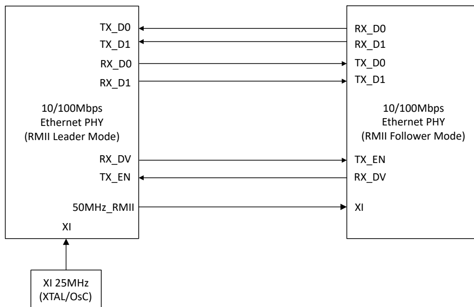
图 8-6. RMII 中继器模式：主-从
