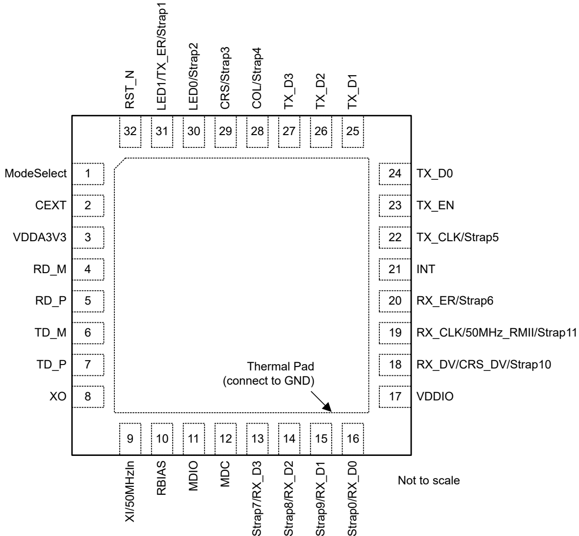
图 6-1. RHB 封装 32 引脚 QFN (俯视图)
