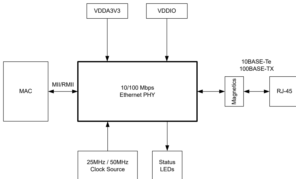
图 9-1. DP83826Ax 典型应用
