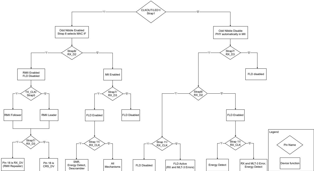
图 8-13. 增强型自动加载流程图
