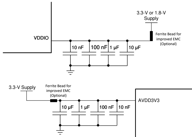
图 9-6. 电源去耦建议
