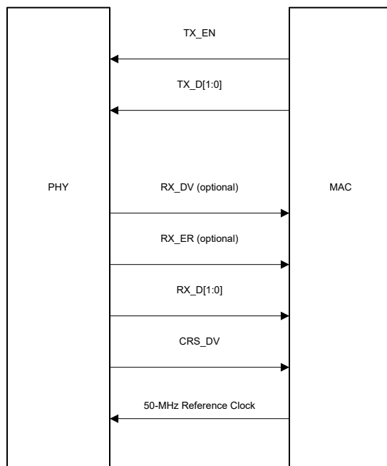
图 8-4. 使用来自 MAC 的 50MHz 时钟的 RMII 从模式信令
