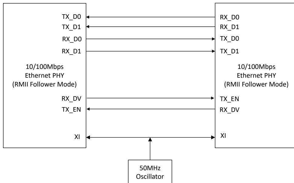
图 8-7. RMII 中继器模式：从-从
