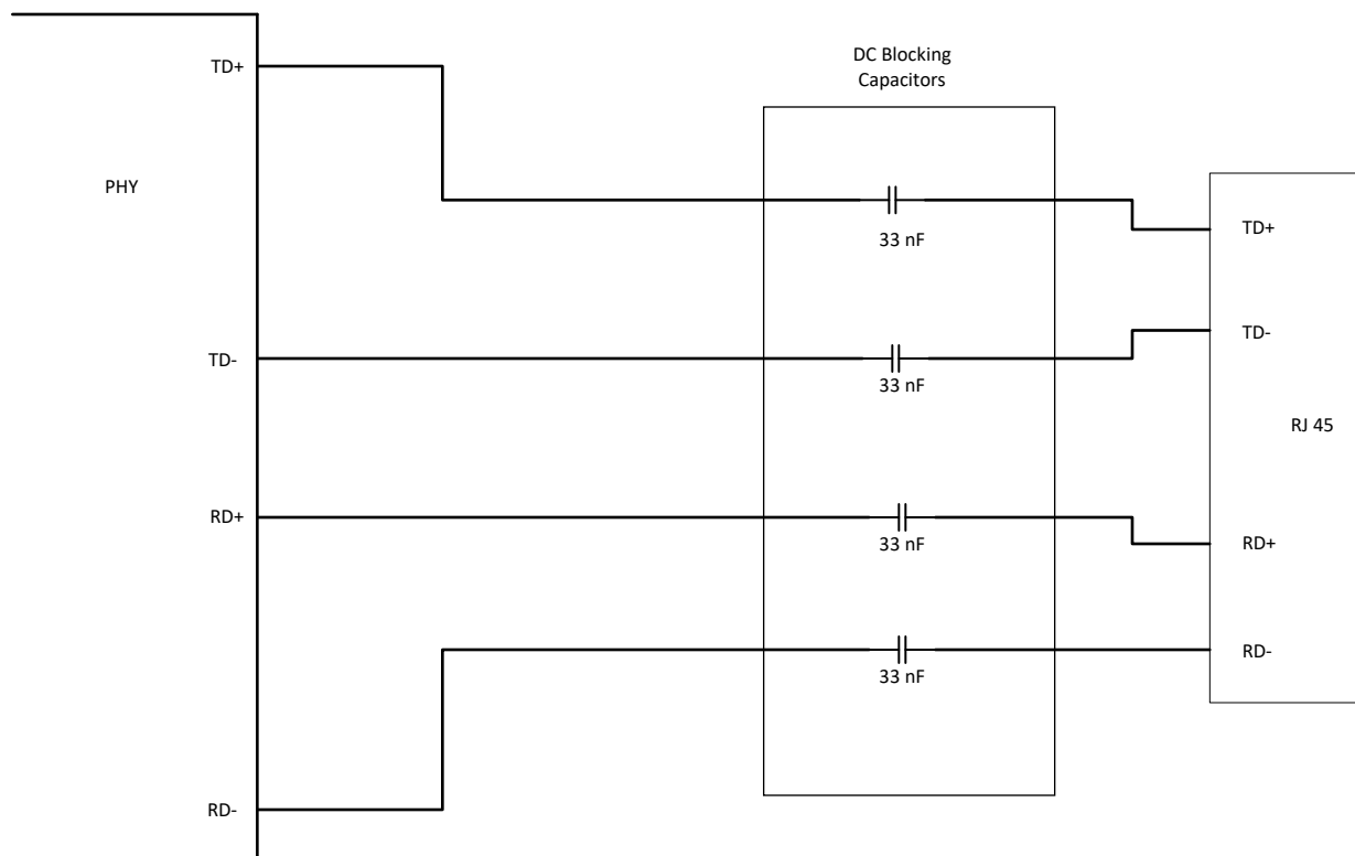
图 9-3. 无变压器直流阻断配置
