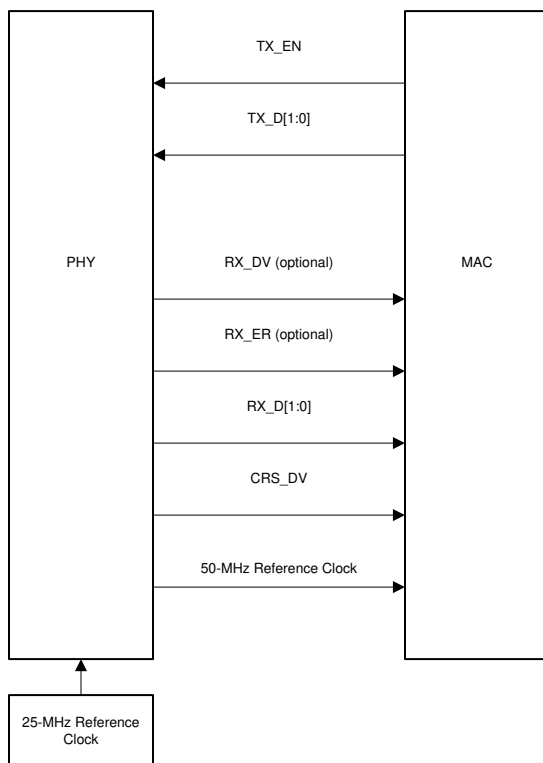
图 8-5. RMII 主信令
