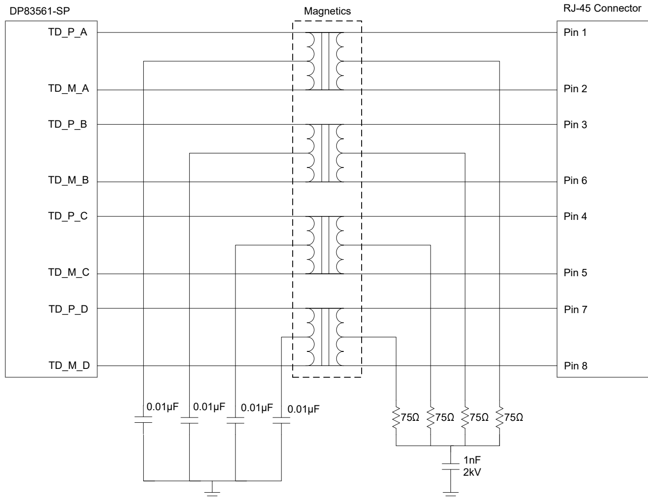
图 8-3. Magnetics Connection
