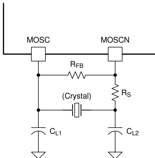
图 9-4. Crystal Oscillator Configuration
