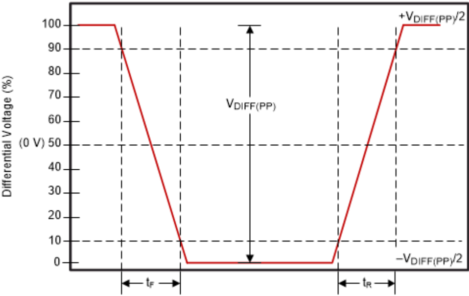
图 6-15. DMD 低速差分时序参数
