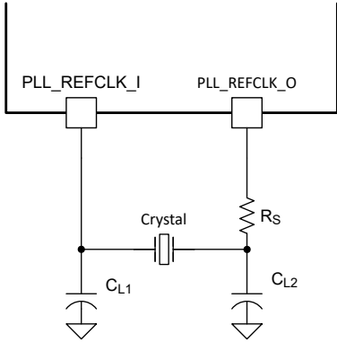
图 8-1. 晶体所需的分立式元件
