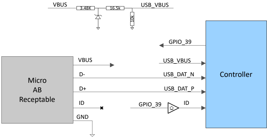
图 5-5. DLPC8445 和 DLPC8445V 控制器的 USB 示例
