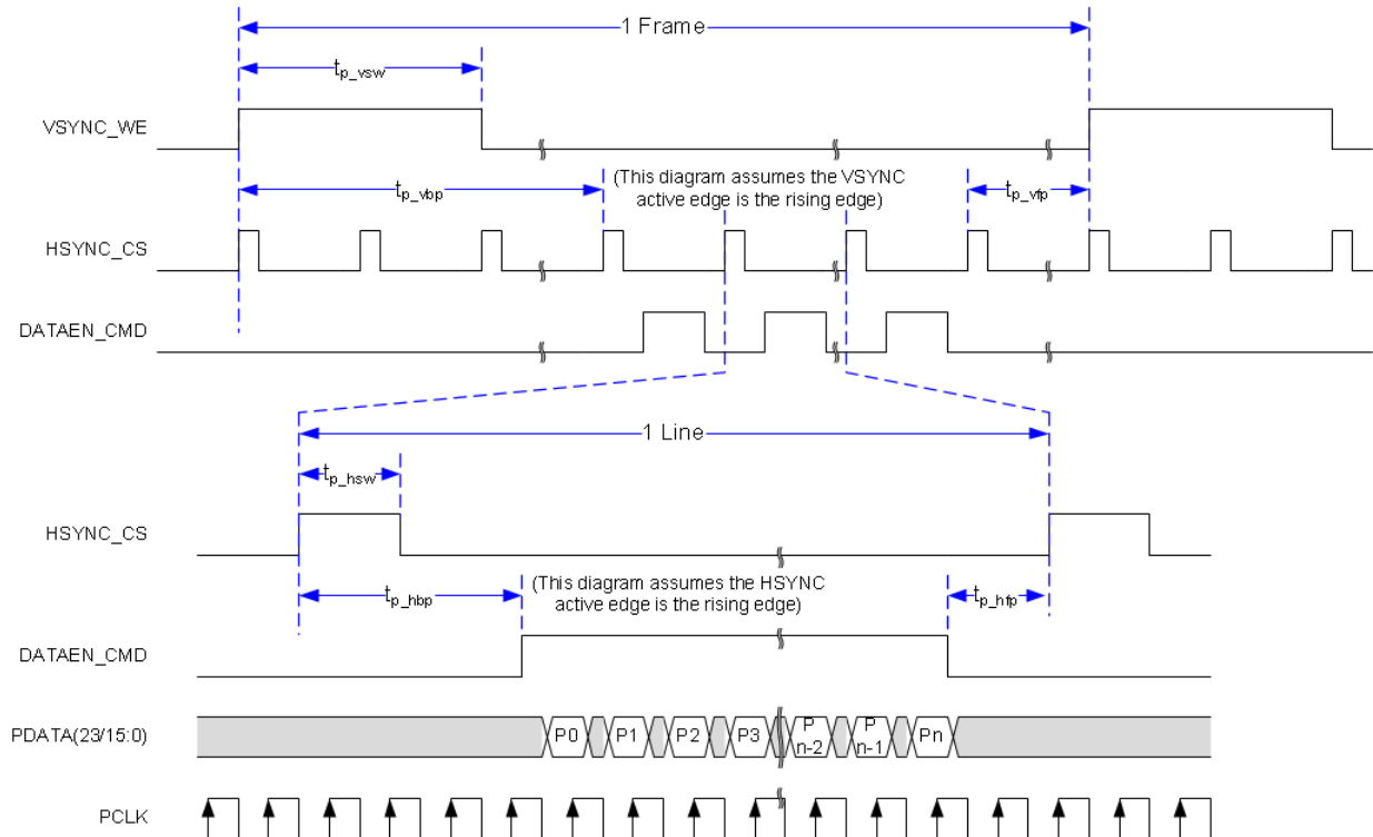
图 5-10. 源帧时序
