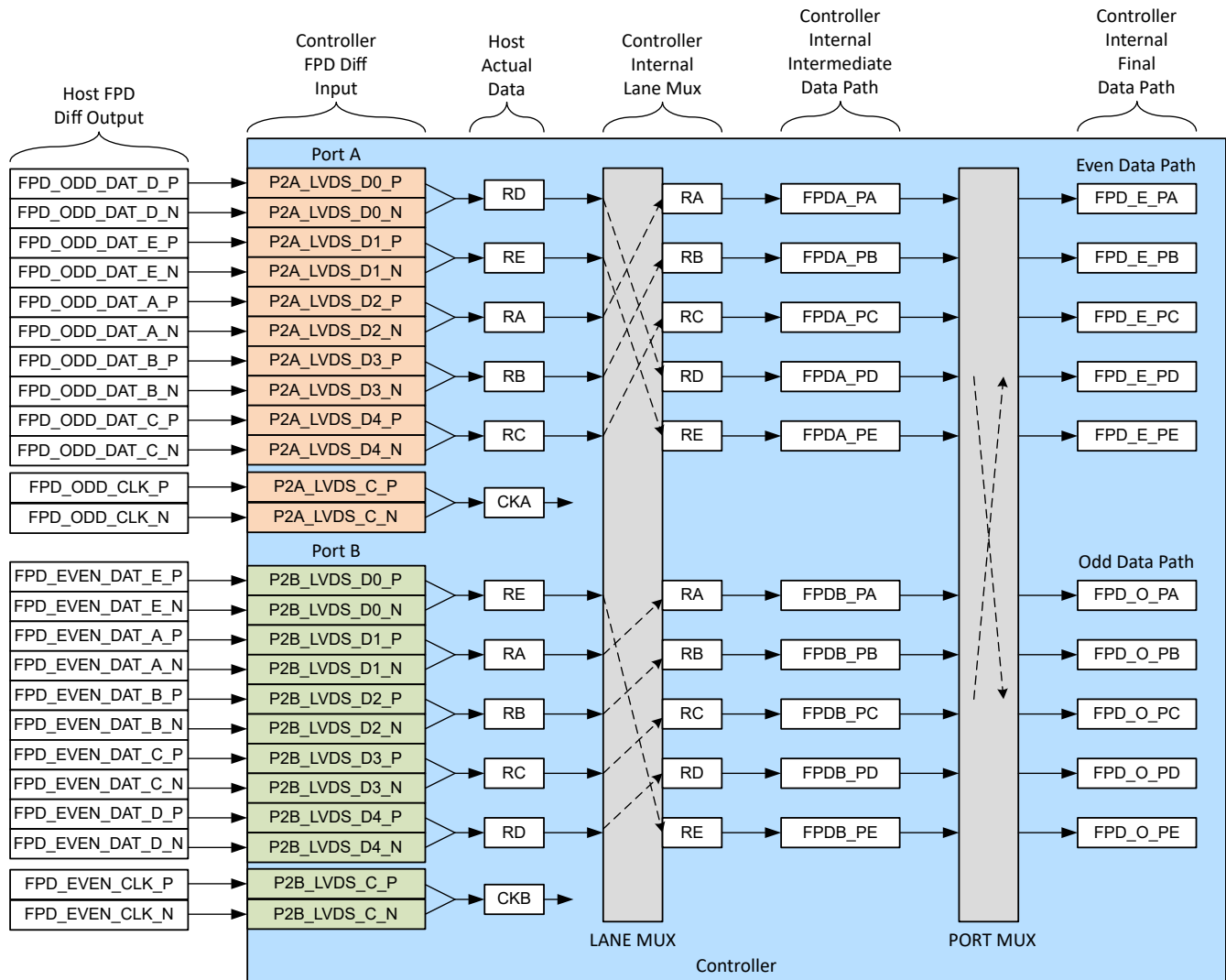
图 7-3. 备用 FPD-Link 端口通道映射示例
