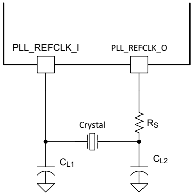
图 9-1. 晶体所需的分立式元件
