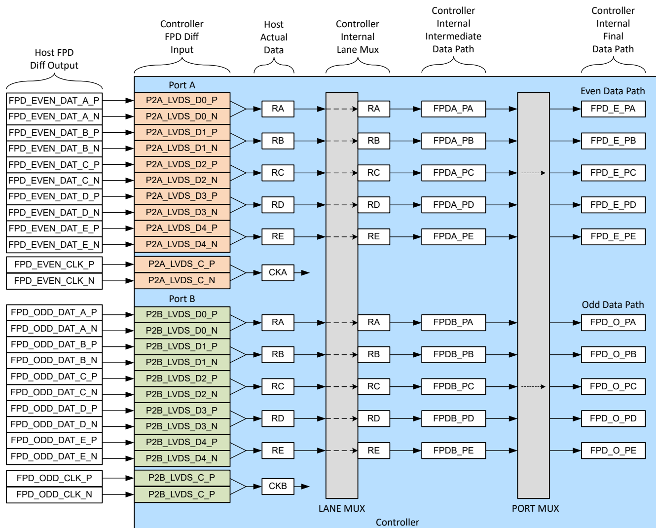
图 7-2. 典型 FPD-Link 端口通道映射示例
