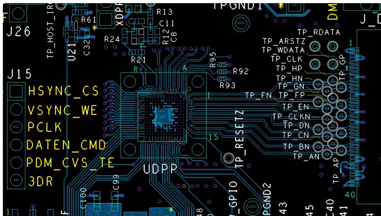
图 10-3. Layout Recommendation
