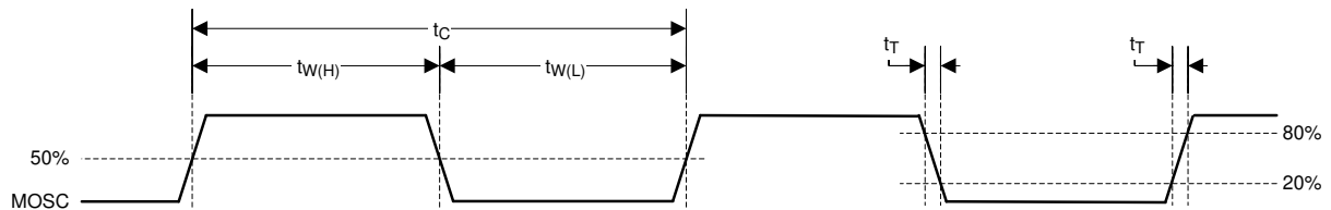
图 5-5. System Oscillators
