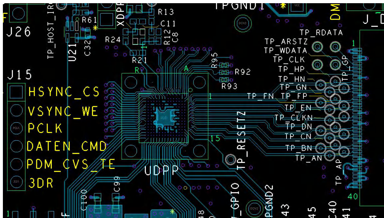
图 9-3. Layout Recommendation
