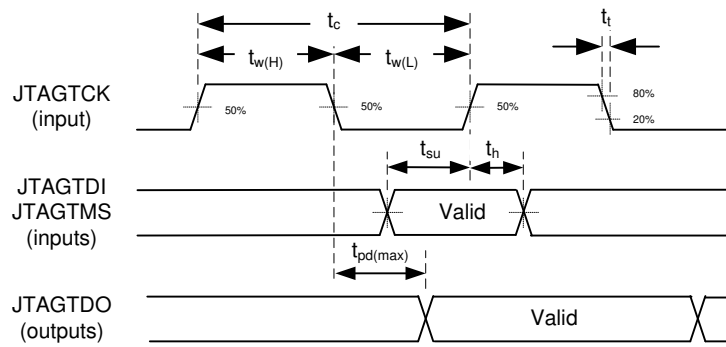
图 6-7. JTAG Interface Timing
