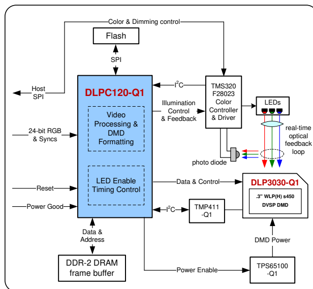
典型系统图
