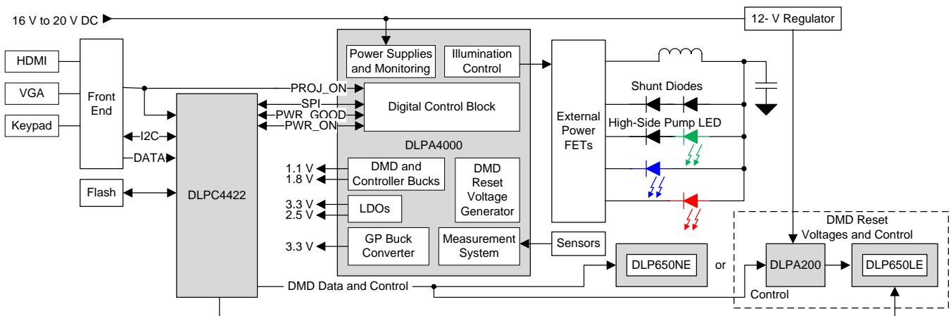
系统方框图
