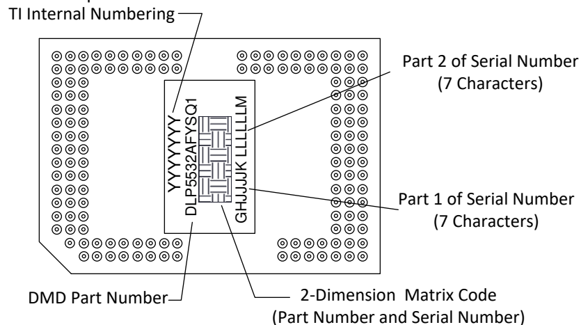
图 11-2. DMD Marking
