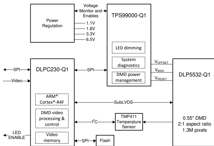
DLP5532-Q1 TI DLP® 芯片组系统方框图
