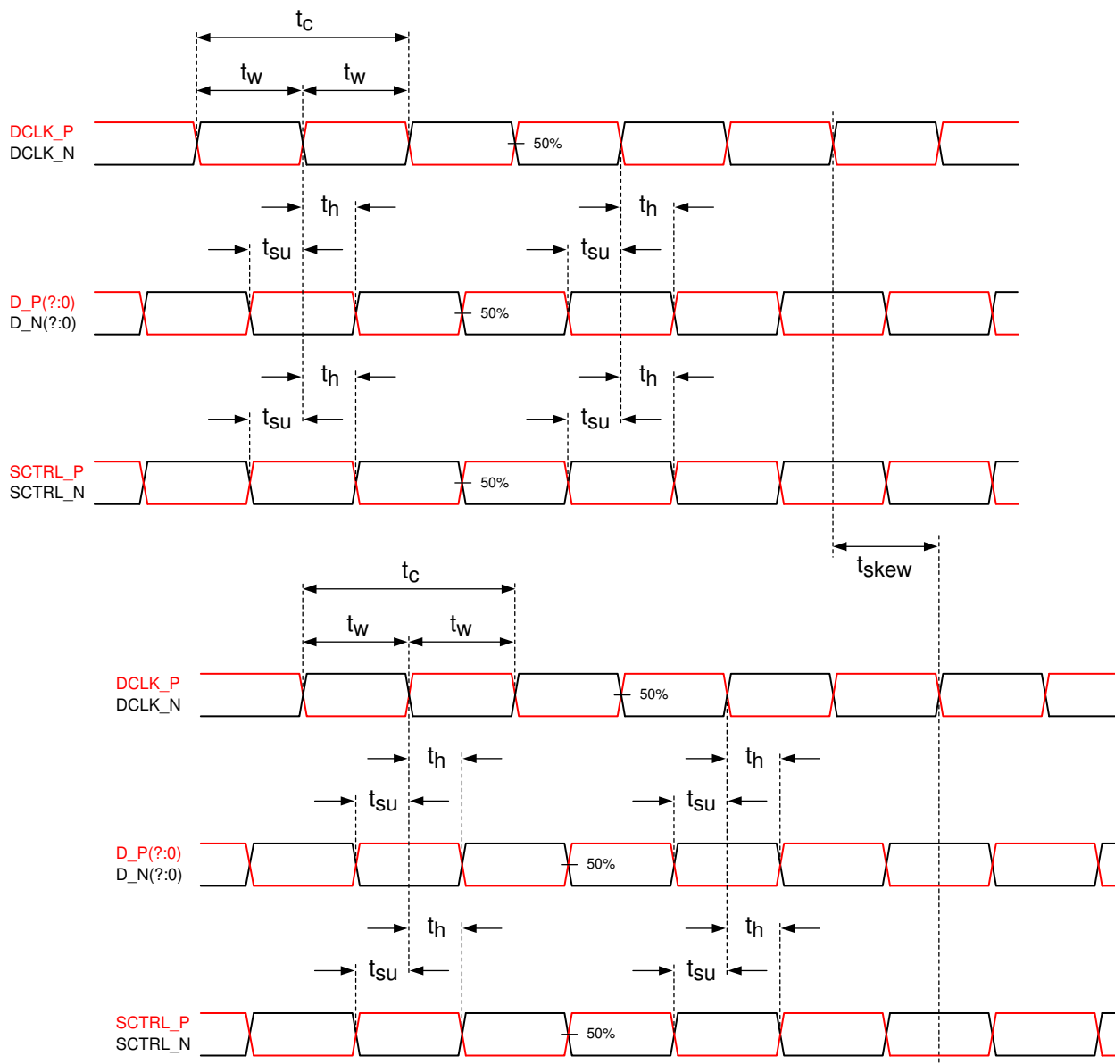
图 5-6. Timing Requirements
