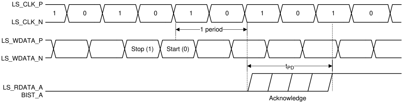
图 5-3. 开关特性
