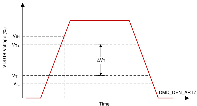
图 5-8. LVCMOS Input Hysteresis
