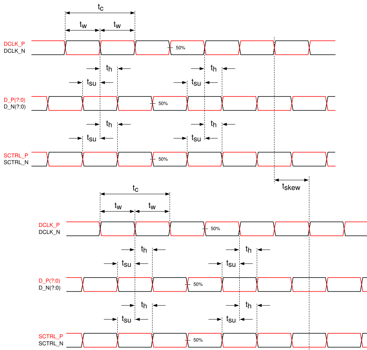
图 5-6. Timing Requirements
