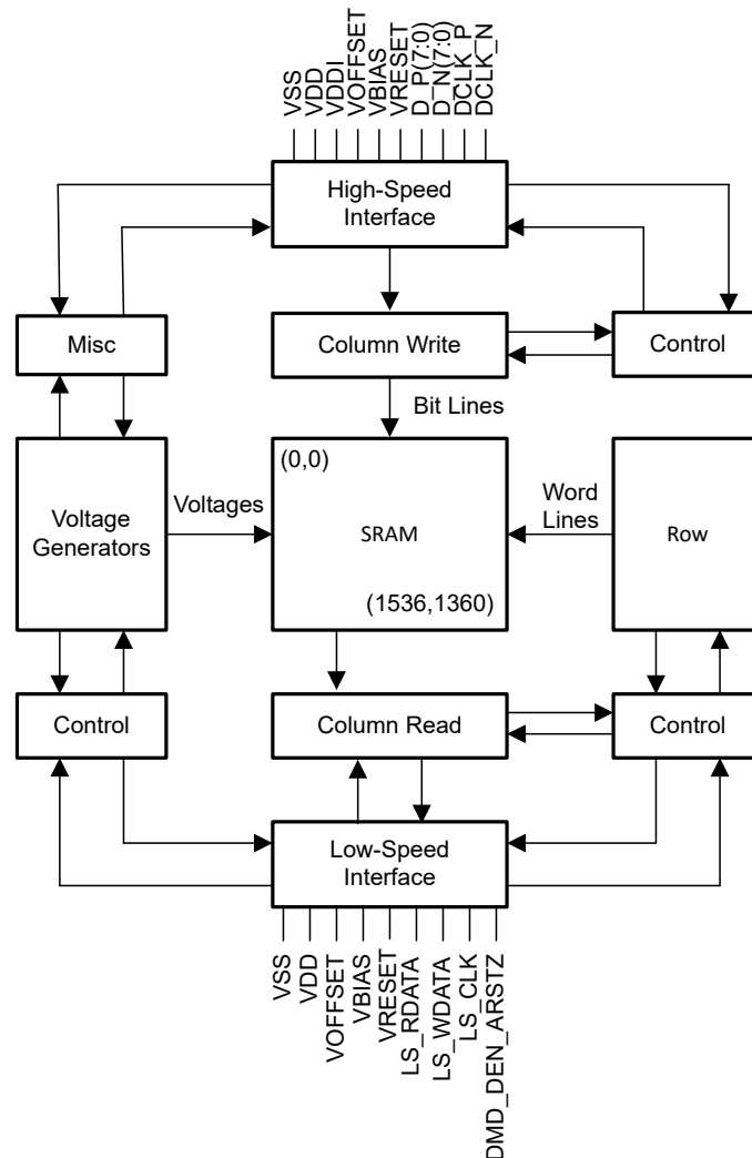
图 6-1. 功能方框图
