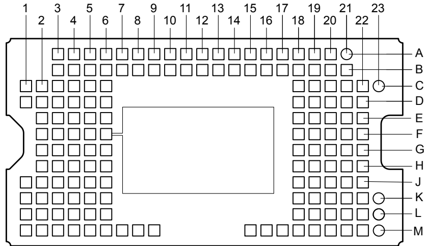
图 4-1. FSB 封装，154 引脚 LGA (底视图)
