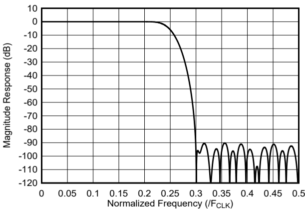
图 7-14. 2 倍内插滤波器响应
