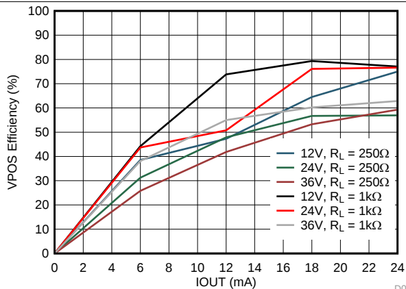
图 79. IOU T VPOS Efficiency
