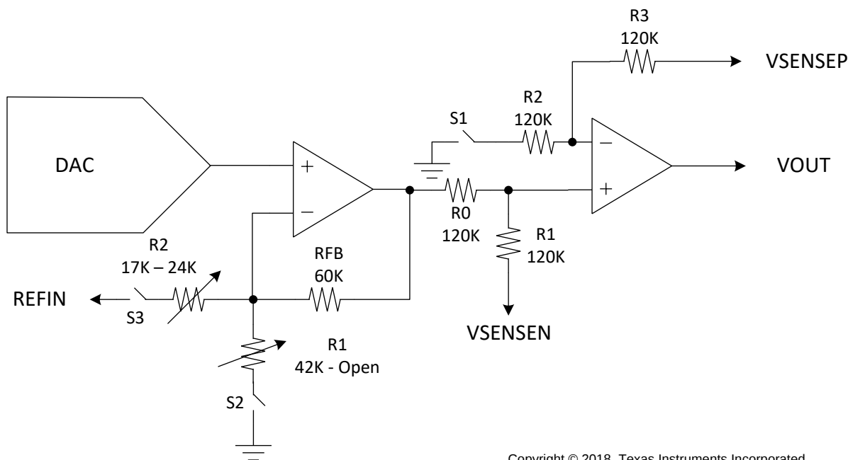
图 98. Voltage Output
