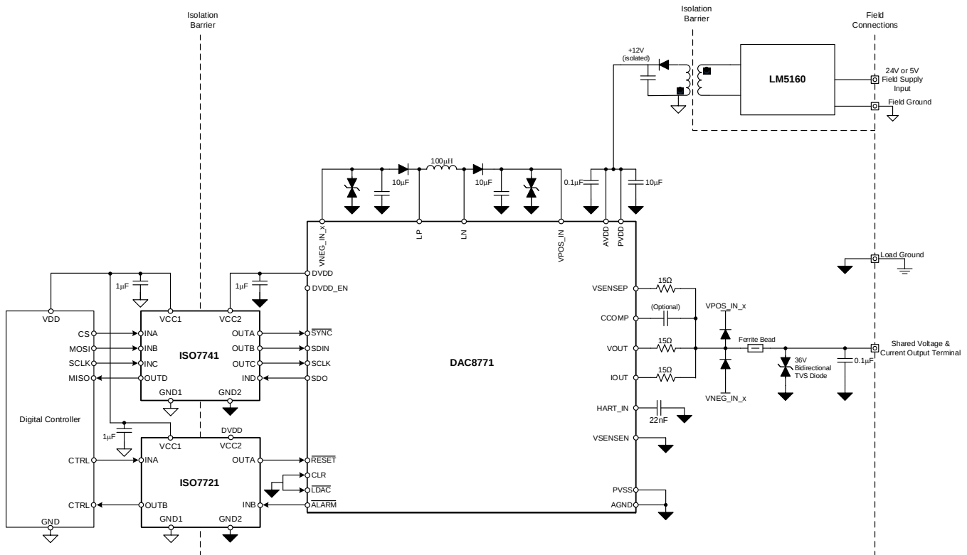
图 125. DAC8771 在隔离单通道 PLC AO 模块
