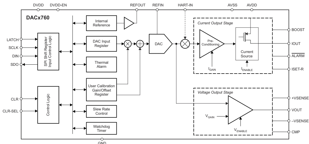
方框图
