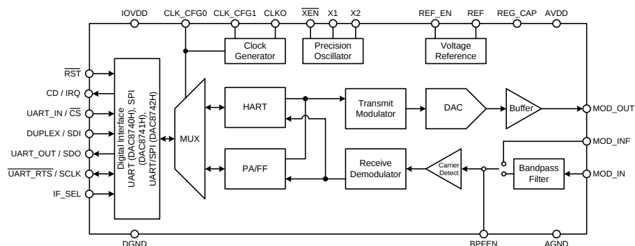
简化原理图
