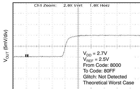
Figure 44. Glitch Energy: Rising Edge
