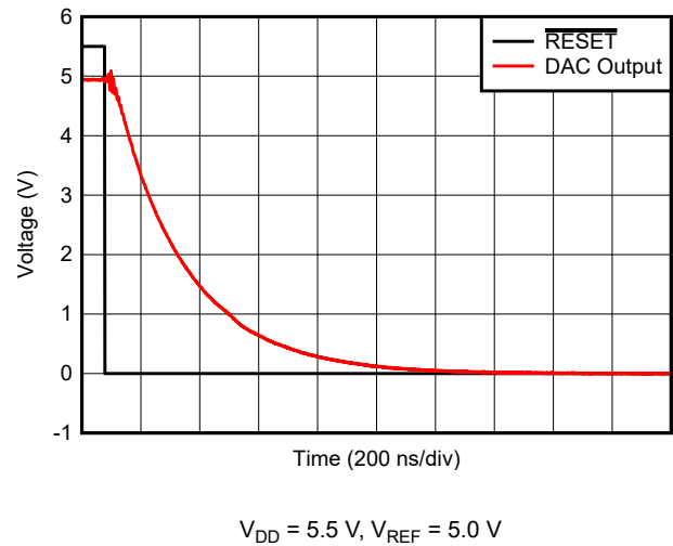
图 6-25. RESET Response
