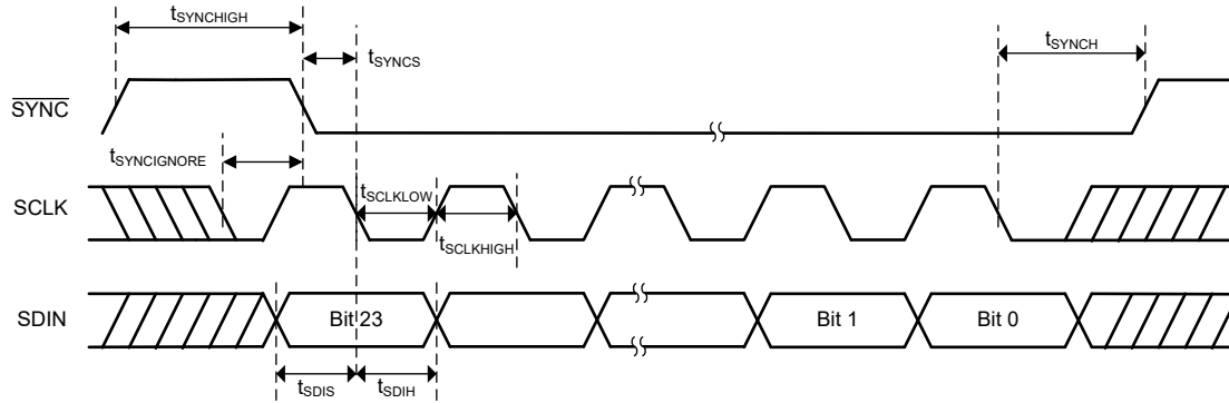
图 6-1. Timing Diagram
