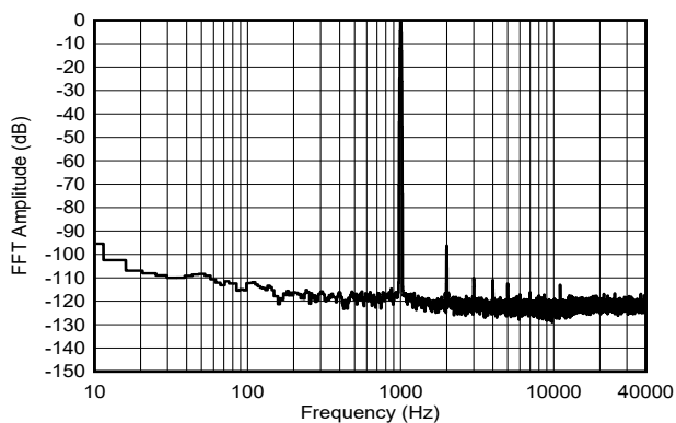
图 8-3. FFT Amplitude vs Frequency
