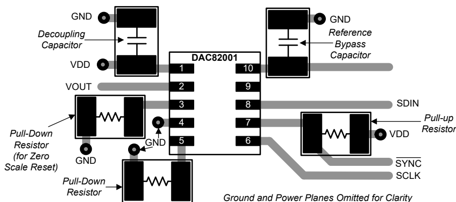
图 8-8. Layout Example
