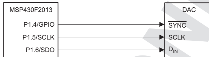
图 100. DAC756x-Q1, DAC816x-Q1, or DAC856x-Q1 Device to MSP430 Interface
