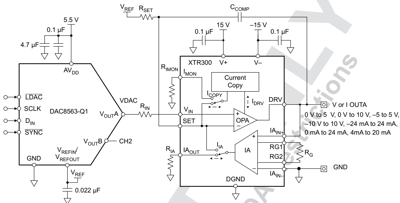
图 96. DAC8563-Q1 and XTR300 Discrete Analog Output Module
