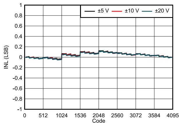
图 7-9. DAC61404 INL vs Digital Input Code (Bipolar Outputs)
