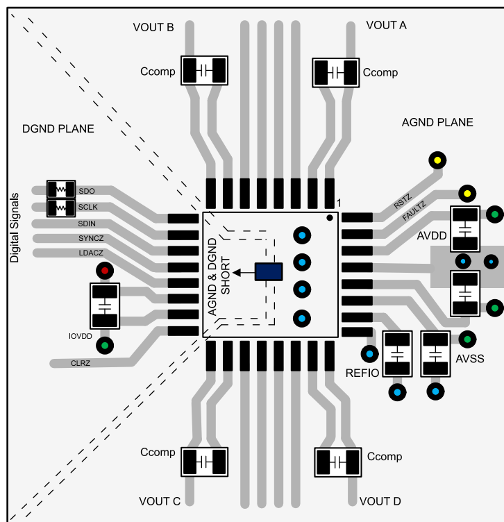
图 11-1. Layout Example
