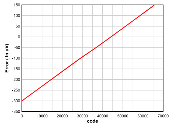
图 9-3. Output Error vs DAC Code
