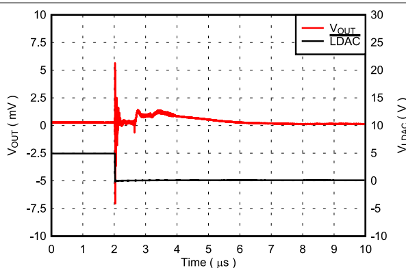
图 7-37. Glitch Impulse, 1 LSB Step, Falling Edge
