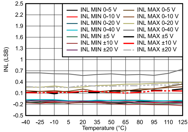
图 7-15. DAC81404 INL vs Temperature
