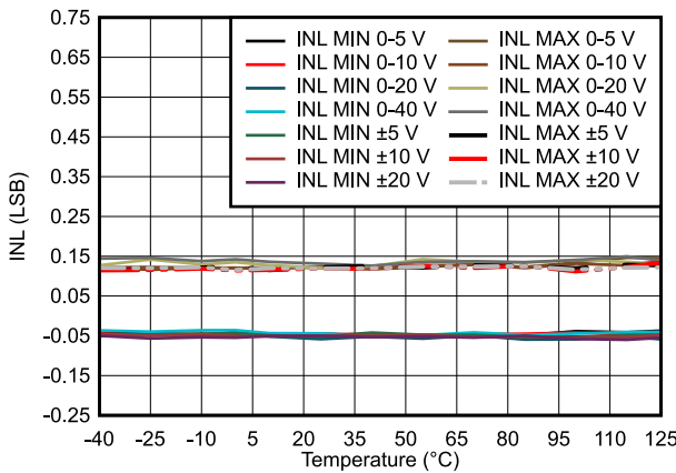
图 7-17. DAC61404 INL vs Temperature
