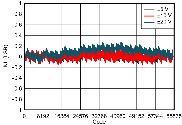
图 7-3. DAC81404 INL vs Digital Input Code (Bipolar Outputs)
