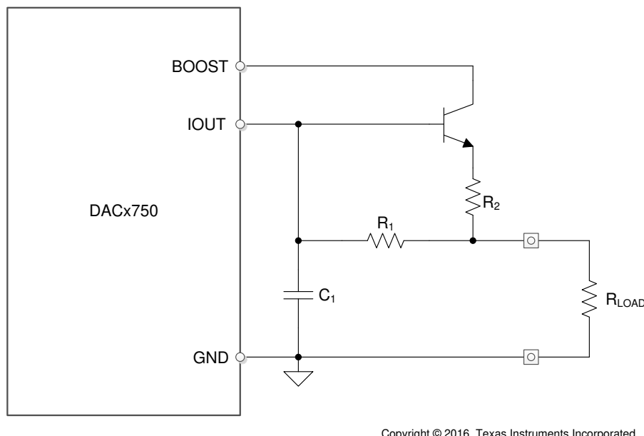
图 8-5. Boost Mode Configuration
