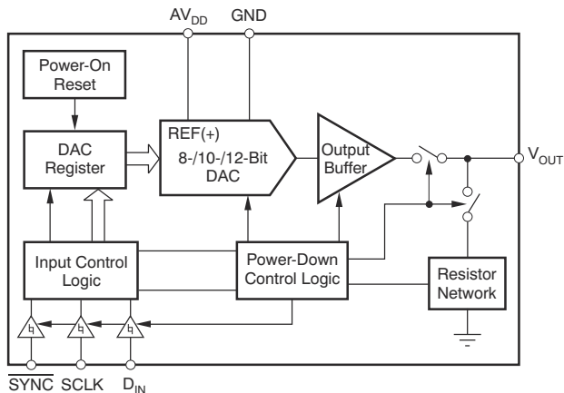
简化原理图
