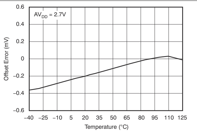
图 7-53. Offset Error vs Temperature
