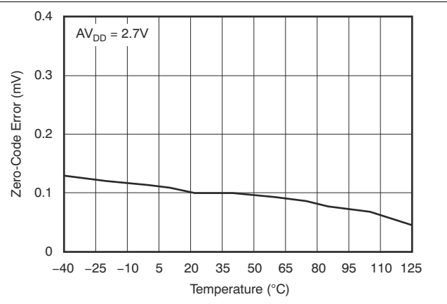
图 7-51. Zero-Code Error vs Temperature
