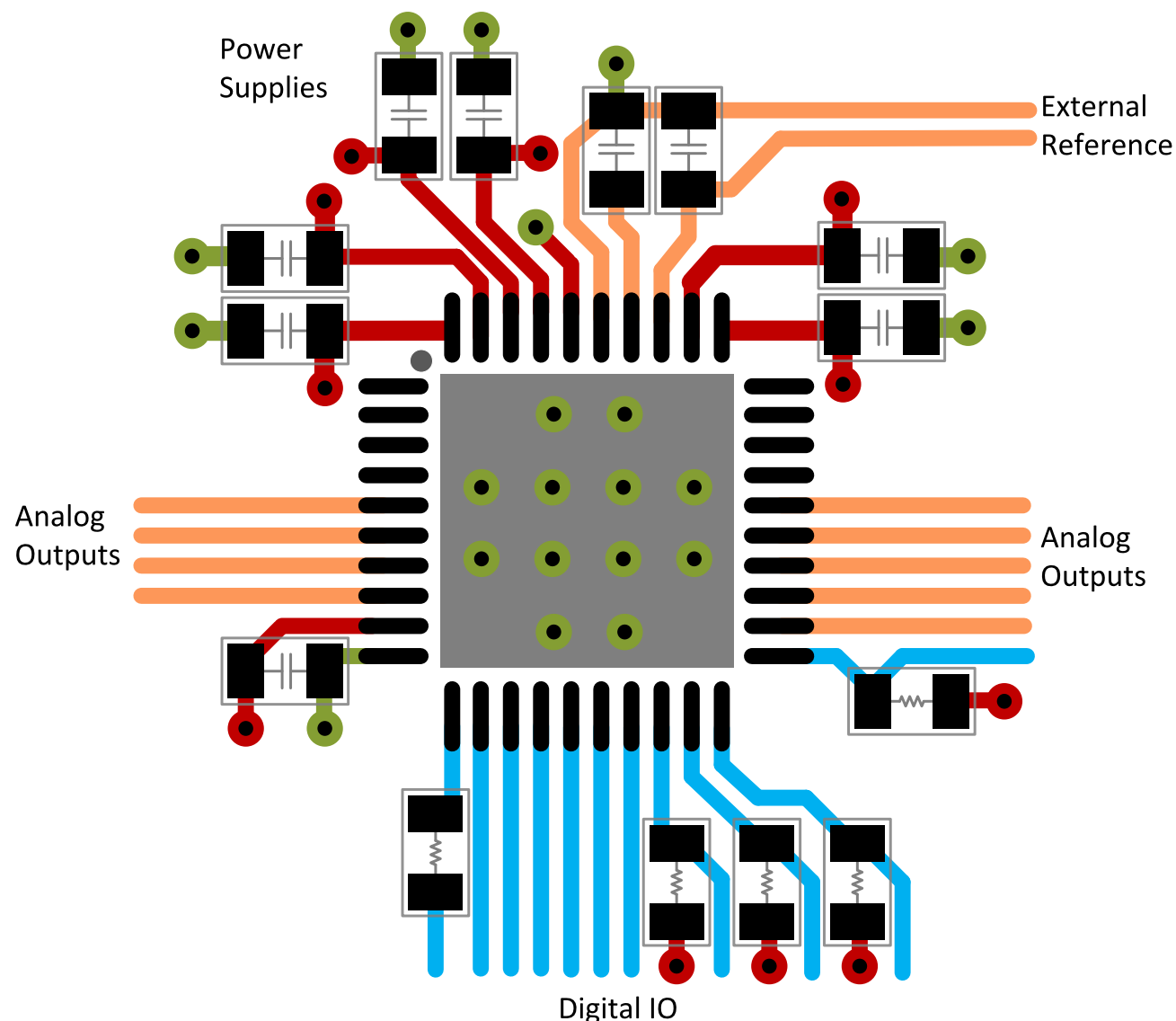
图 70. Example Layout
