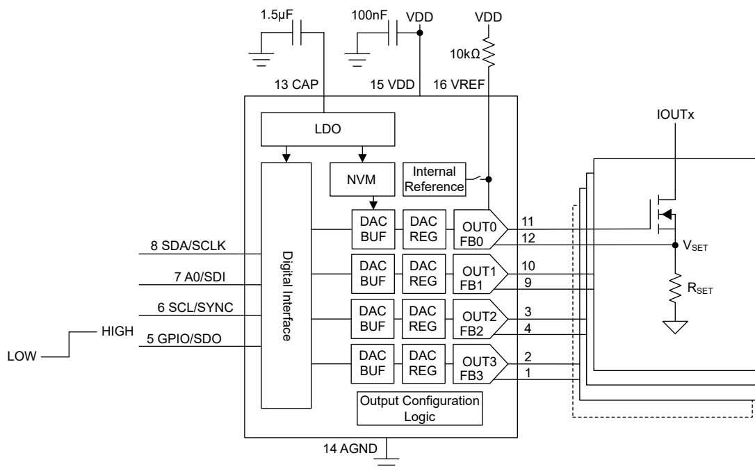
图 8-1. Current Source
