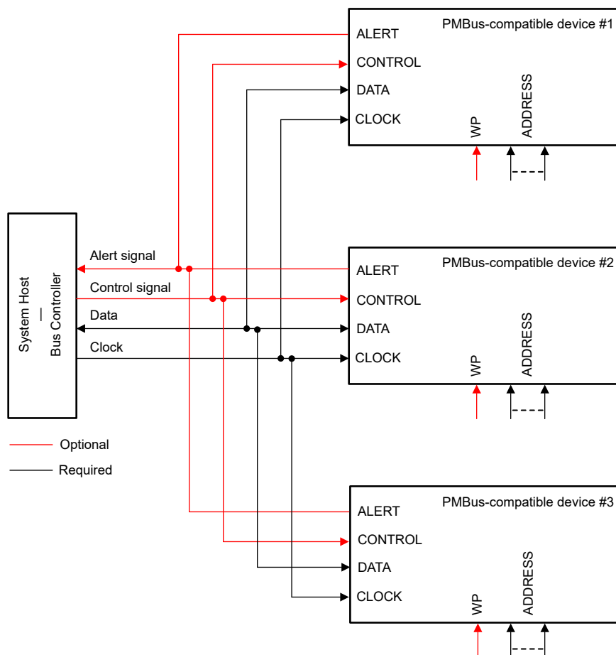
图 7-11. PMBus Connections
