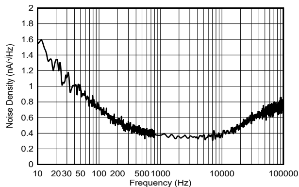
图 6-49. Current Output Noise Density
